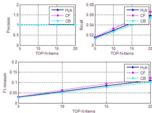
Figure 4.14: Performance de la recommandation basée prédiction
