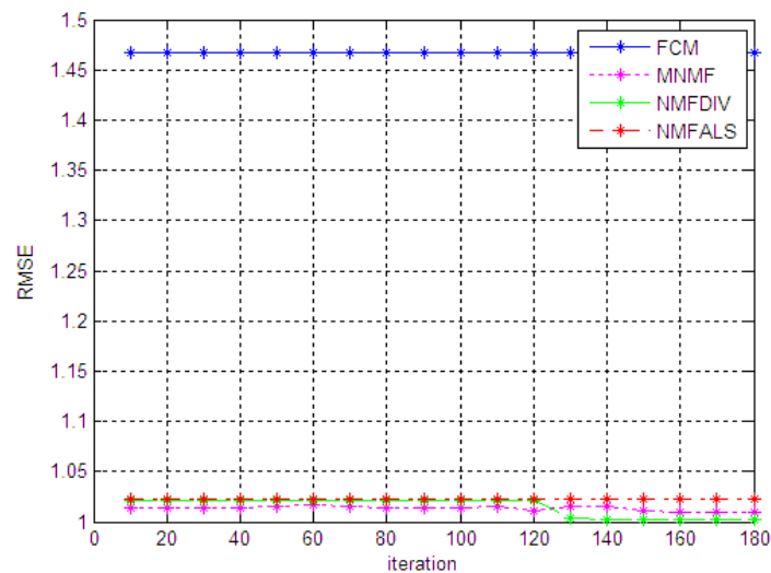
Figure 4.4: RMSE pour différents algorithmes de clustering (petite valeur, meilleure performance)
