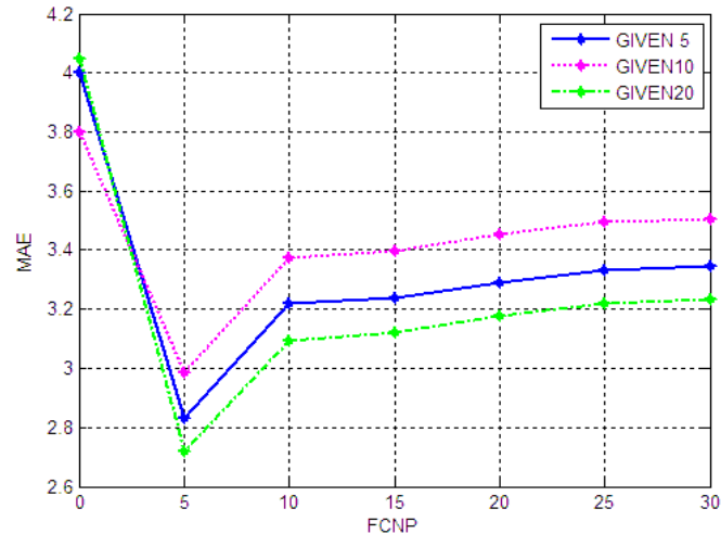
Figure 4.5: Valeur optimale des plus proches clusters flous
