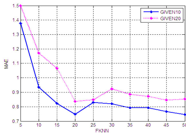
Figure 4.6: Valeur optimale des plus proches voisins flous
