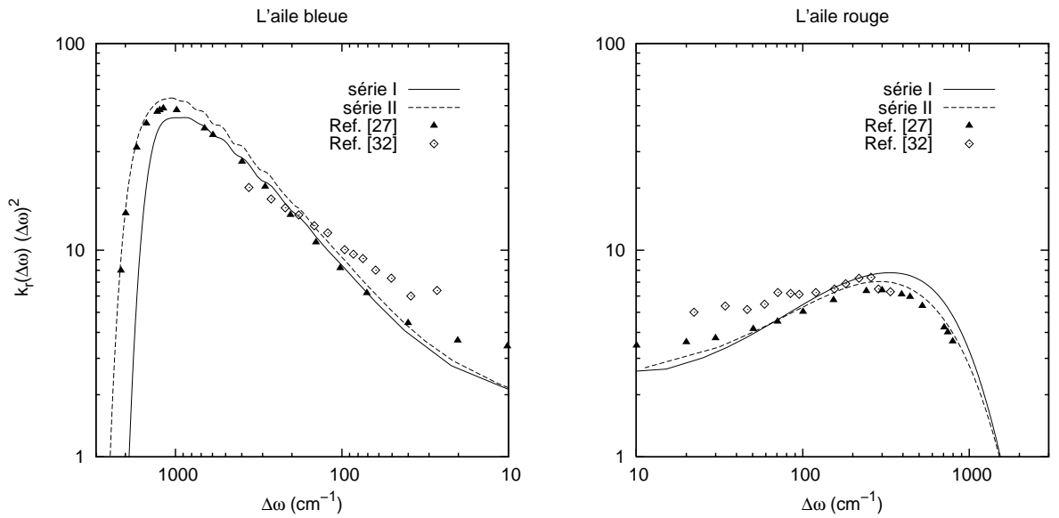
FIG. 4-6 – Coefficients d'absorption réduits modifiés k_r(\Delta\omega) \times (\Delta\omega)^2 à T = 800 \text{ K} en fonction de \Delta\omega = |\omega - \omega_0| . Nos résultats sont représentés par des lignes continues et en pointillés pour les série I et II, respectivement. Ils sont comparés avec les valeurs théoriques de la Réf. [27] et expérimentales de la Réf. [33].
