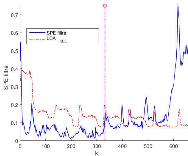
FIGURE 5.16 – SPE filtré pour un défaut dérive affectant le capteur N_{Hainf} de la station réelle.
