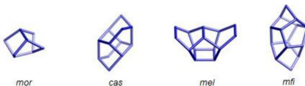
Figure (II.3) : Unités de construction dont l'assemblage régulier est à l'origine du type structural MFI [6]
