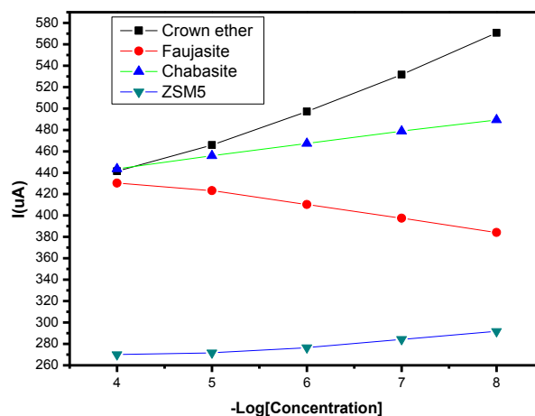
Figure (IV.18) : Effet des teneurs en ionophore de la zéolite sur les capteurs à base de Faujasite, Chabasite, ZSM5, éther de couronne utilisant un plastifiant PEG.
