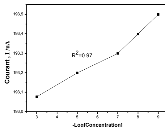
Figure (IV.23) : Voltammogramme à signaux carrés obtenus après injection de différentes concentrations de Gadolinium . Courbe de calibration présentant la
