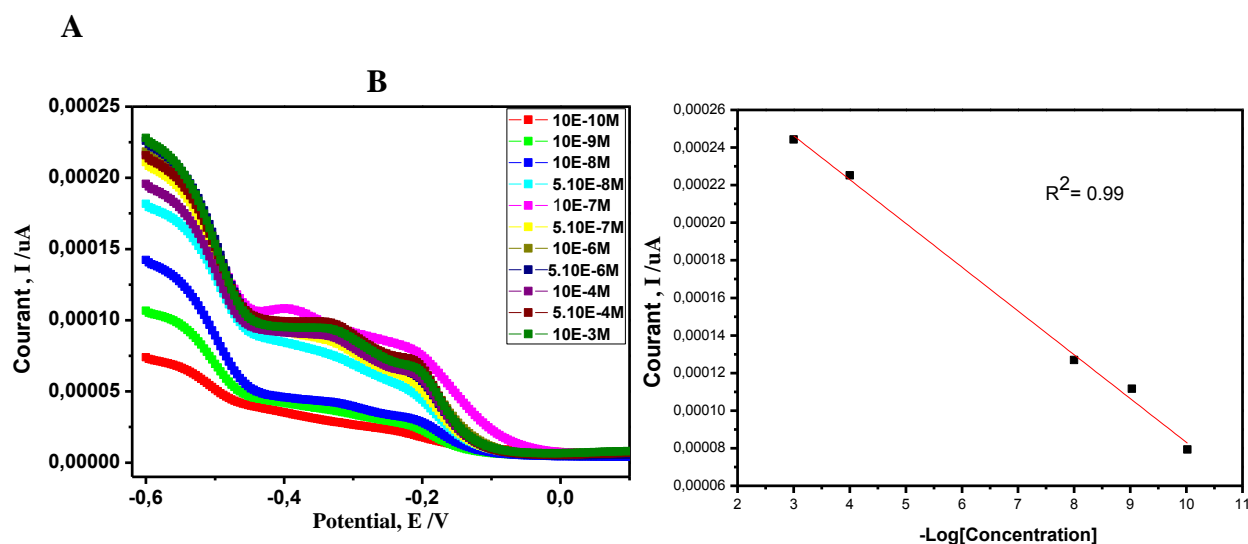
Figure (IV.10) :A. Voltammogrammes à signaux carrés obtenus après injection de différente concentrations de Fe(NO 3 ) 3 B. Courbe de calibration présentant la variation
