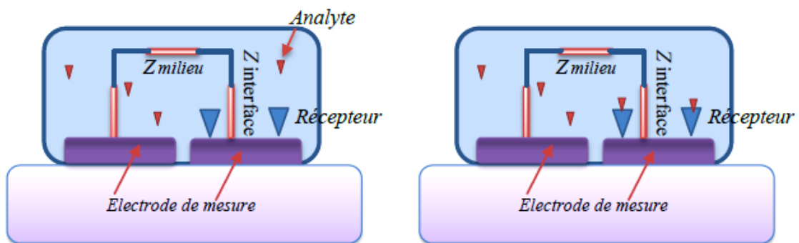
Figure (I.10) : Principe de la transduction conductimétriques.
