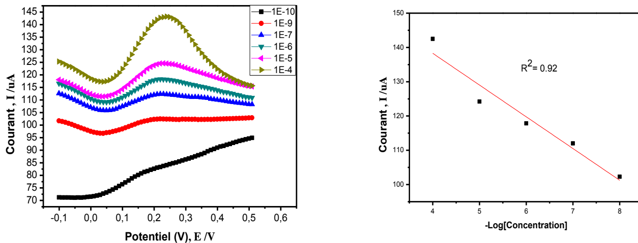
Figure (IV.34) : Voltamogramme à signaux carrés obtenus après injection de différentes concentrations de fer dans la cinquième échantillonne réels. Courbe de calibration présentant la variation de courant des pics d'oxydation en fonction des différentes concentrations de fer en milieu 0.1M NaNO 3 ajuster avec 0.1 M HCl (pH: 2).
