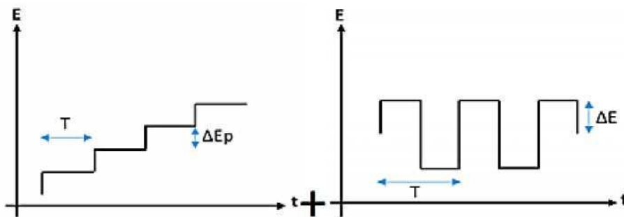
Figure (III.4) : Superposition de la tension carrée symétrique à une tension en escalier
