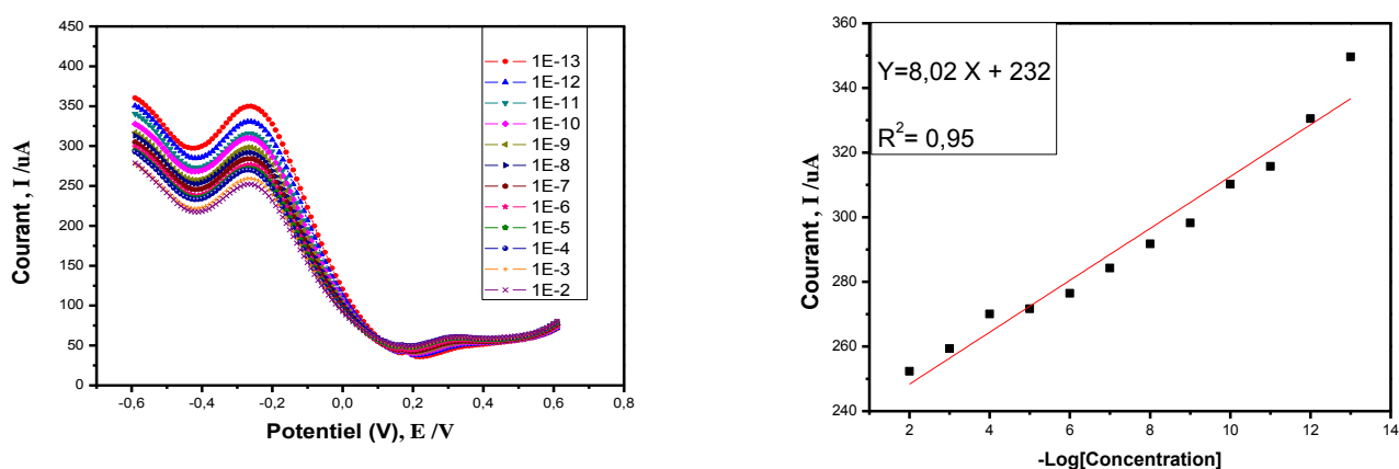
Figure (IV.17) : A. Voltammogrammes à signaux carrés obtenus après injection de différentes concentrations de Fe (NO 3 ) avec la membrane d'ionophore ZSM-5. B. Courbe de calibration présentant la variation de courant des pics d'oxydation en fonction des différentes concentrations de fer en milieu 0.1M NaNO 3 ajuster avec 0.1 M HCl (pH: 2).
