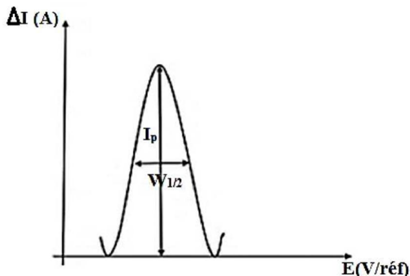
Figure (III.7) : Voltammogramme à signaux carré représentatif des courbes obtenues avec la méthode
