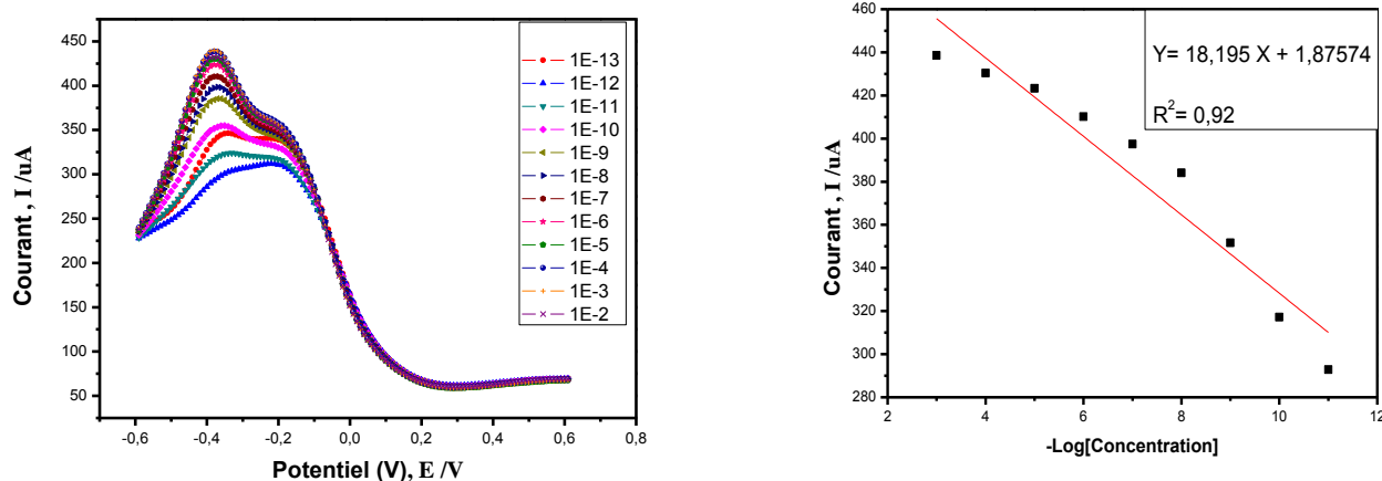
Figure (IV.15) :A. Voltammogrammes à signaux carrés obtenus après injection de différentes concentrations de Fe (NO 3 ) avec la membrane d'ionophore (FAUJASITE (FAU)). B. Courbe de calibration présentant la variation de courant des pics
