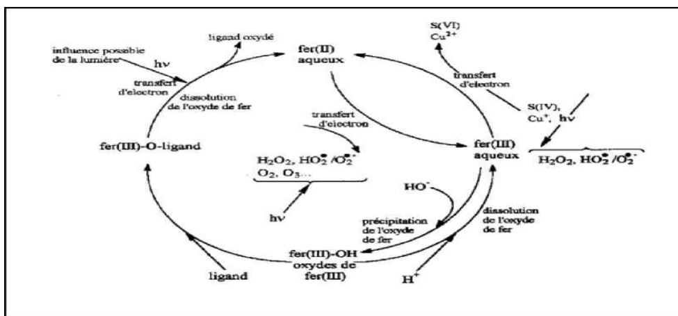
Figure (I.1) : Cycle du Fe dans l'eau en contact avec l'air selon (Behra et al;1990) [20].
