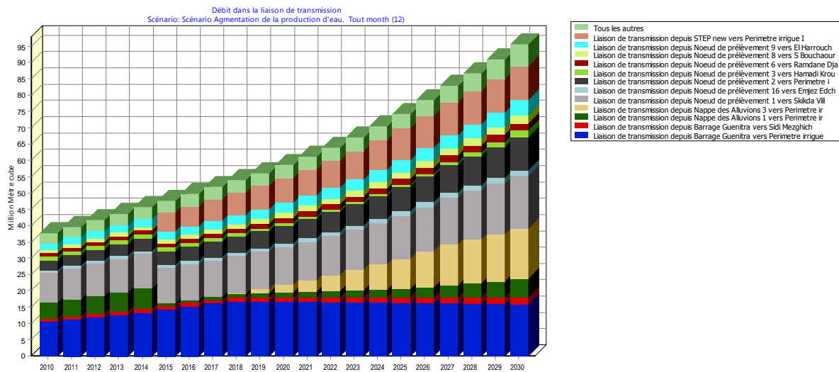
Figure VI.46. Apports de la STEP et des autres sources à l’approvisionnement. -Scénario 4 : Augmentation de la production de l’eau (2011-2030)-
