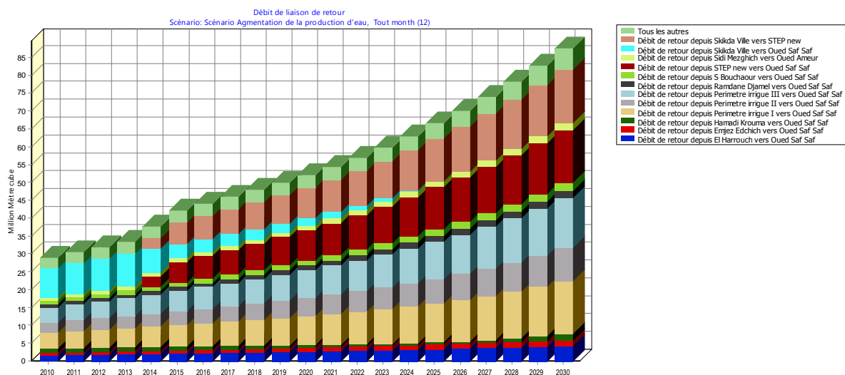
Figure VI.47. Débits de retour des nouvelles source d’approvisionnement. -Scénario 4 : Augmentation de la production de l’eau (2011-2030)-
