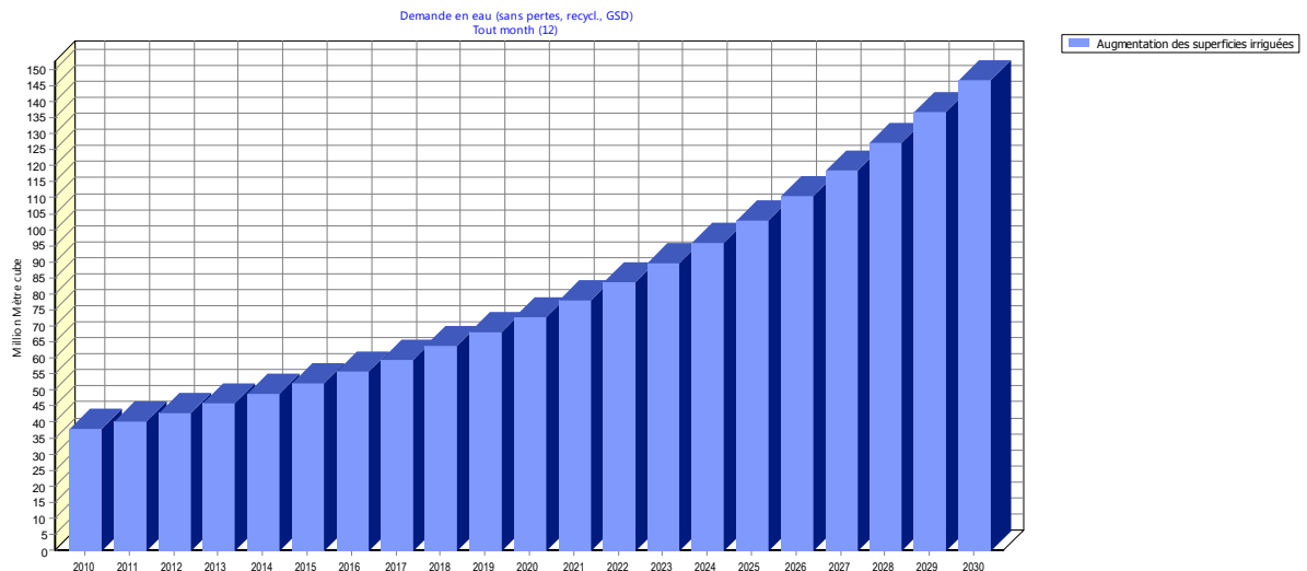
Figure VI.35. Evolution de la demande en eau globale dans le bassin versant du Saf-Saf. -Scénario 3 : Augmentation des superficies irriguées (2011-2030)-
