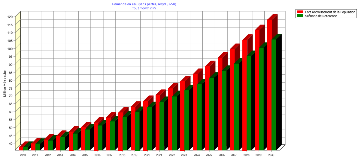
Figure VI.30. L’effet du fort accroissement de la population sur la demande en eau dans le bassin du Saf-Saf. 2011-2030 (en Mm 3 )
