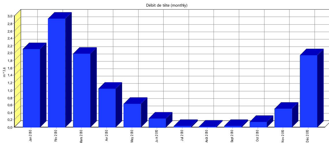
Figure VI.13. Débit de tête de l'oued Saf-Saf (station de Khemakhème). -Compte d'état actuel, 2010-
