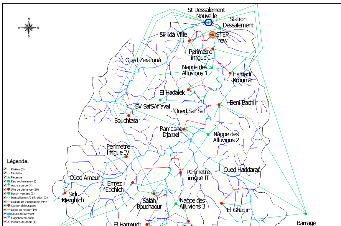
Figure VI.42. Schéma hydraulique projeté de l'aval du bassin du Saf-Saf. -Scénario 4 : Augmentation de la production de l'eau (2011-2030)-
