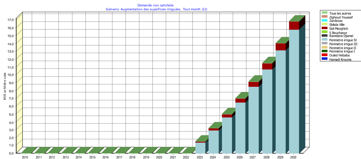
Figure VI.37. Demande en eau non satisfaite dans le bassin versant du Saf-Saf. -Scénario 3 : Augmentation des superficies irriguées (2011-2030)-
