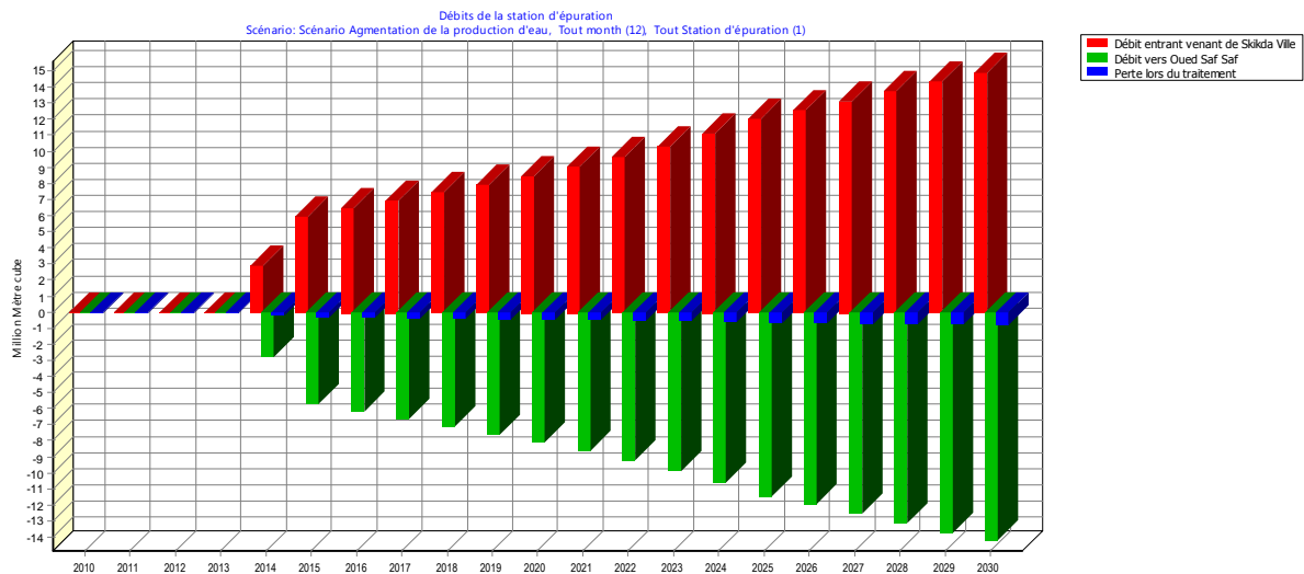
Figure VI.41. Débits entrants et sortants de la station d'épuration. -Scénario 4 : Augmentation de la production de l'eau (2011-2030)-
