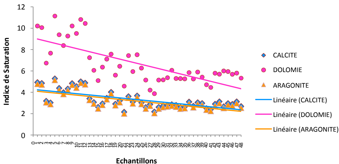
Figure IV.44. Evolution des minéraux carbonatés dans les eaux de surface .
