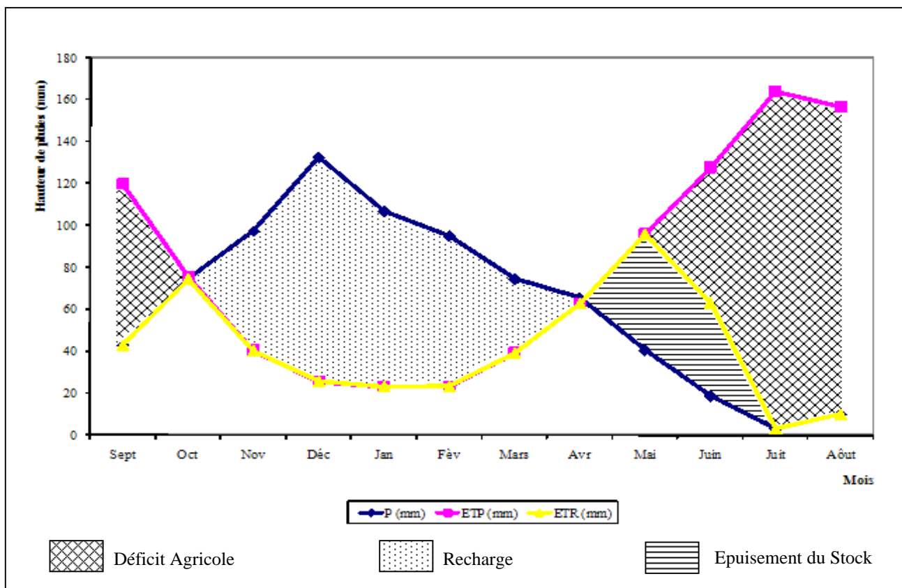
Figure II.10. Représentation graphique du bilan d'eau selon la méthode de C.W. Thornthwaite de la station de Skikda (1970/71-2011/12).
