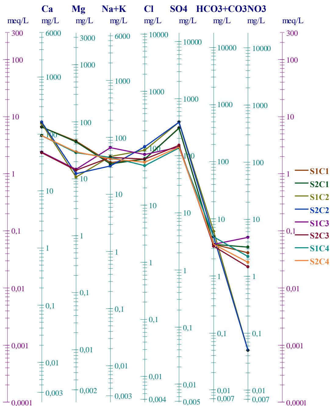
Figure IV.21. Représentation graphique des faciès chimiques des eaux de surface en amont du bassin sur le diagramme de Schëoller-Berkaloff (2012-2013).
