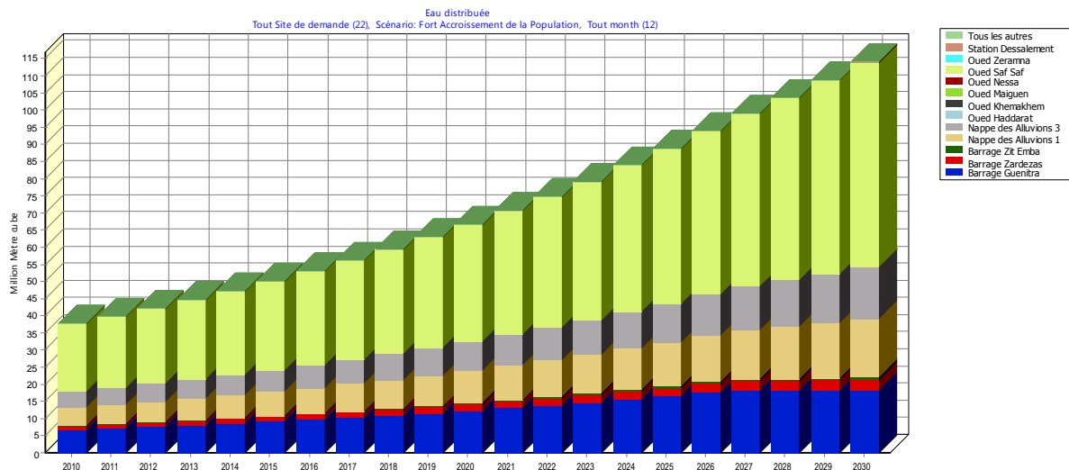
Figure VI.31. Eau distribuée dans le bassin versant du Saf-Saf. - Scénario 2 : Fort accroissement de la population (2011-2030)-
