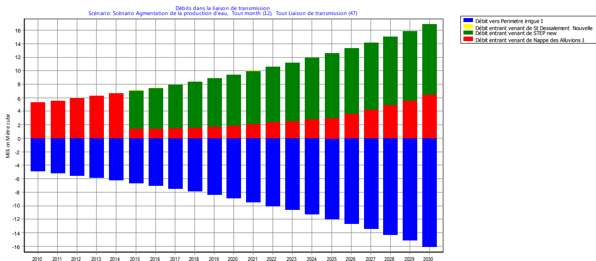
Figure VI.45. Débits entrants à partir des nouvelles sources d'alimentation.
