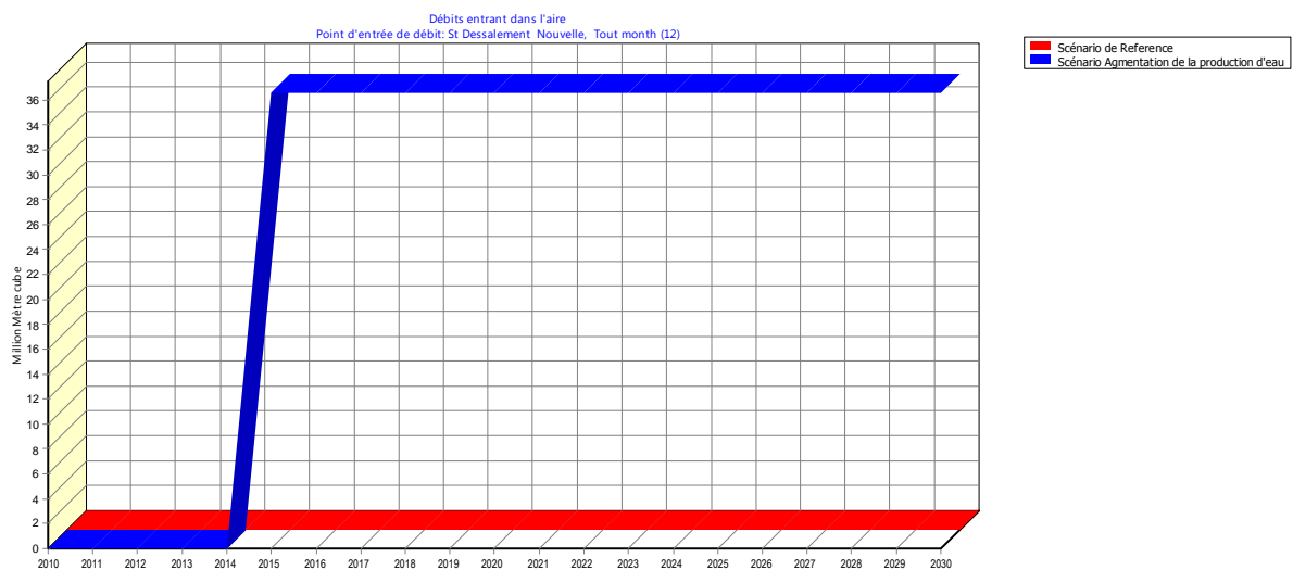
Figure VI.38. Evolution de la production de la nouvelle station de dessalement de l'eau de mer. -Scénario 4 : Augmentation de la production de l'eau (2011-2030)-
