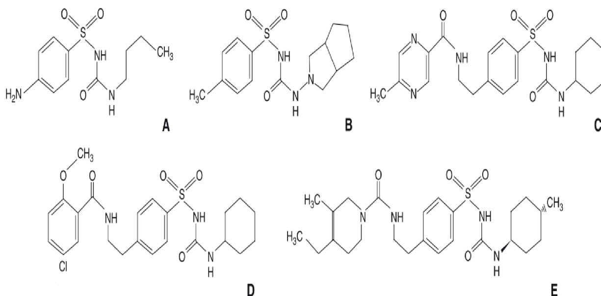
Figure. 15 : Formules chimiques des sulfamides hypoglycémiants. (A). Carbutamide ; (B). Gliclazide ; (C). Glipizide ; (D). Glibenclamide/glyburide ; (E). Glimépiride (Blicklé, 2011).
