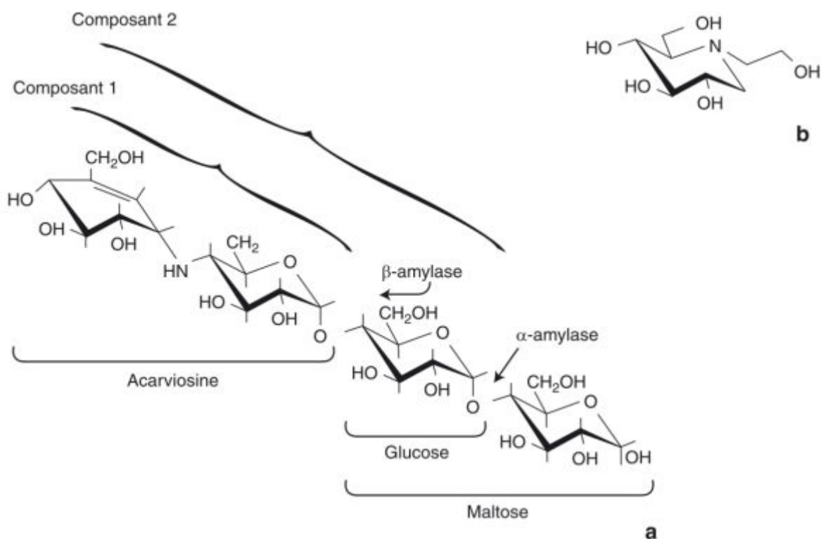
Figure. 8 : Formules chimiques de l'acarbose, de ses produits de dégradation et du miglitol.
