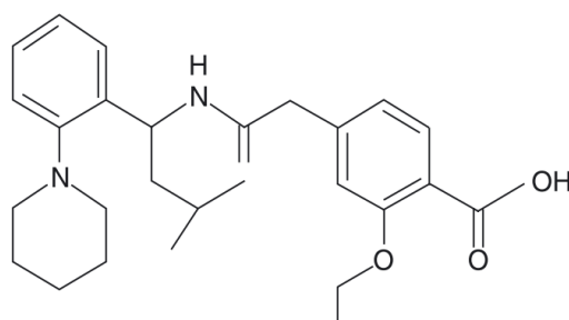
Figure. 5 : Formule chimique du répaglinide (Blicklé, 2011).
