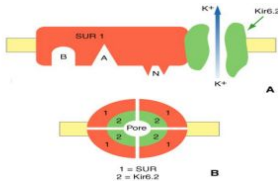
Figure. 17 : Canal potassique sensible à l'ATP : sites de fixation de l'ATP, de sulfonylurées et de glinides (Magan et Ktorza 2005).
