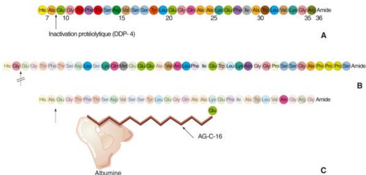
Figure. 10 : Formule chimique du glucagon-like peptide-1 (GLP-1) humain, de l'exénatide et du liraglutide. (A) ; GLP-1 humain, (B) ; Exénatide, (C) ; Liraglutide. DPP-4 : dipeptyl-peptidase-4 (Blicklé, 2011).
