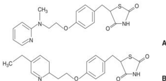
Figure. 7 : Formules chimiques de la rosiglitazone et de la pioglitazone (Blicklé, 2011).
