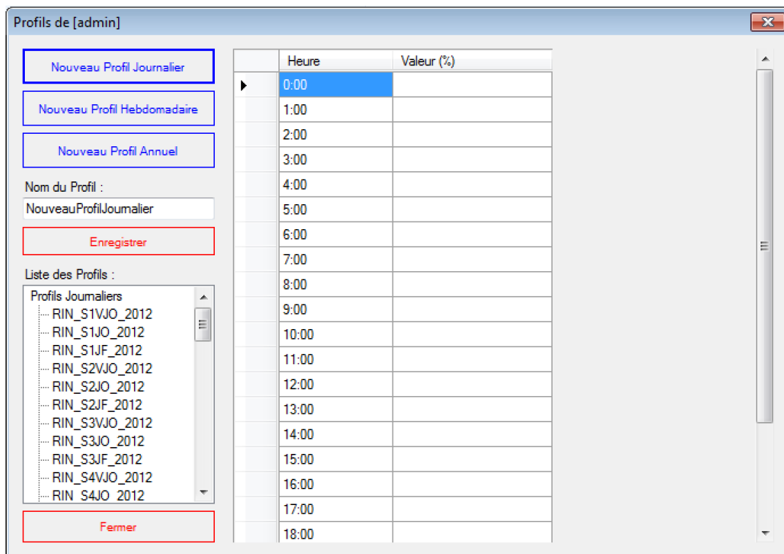
Figure 4.16 – Fenêtre de création et de gestion des profils.
