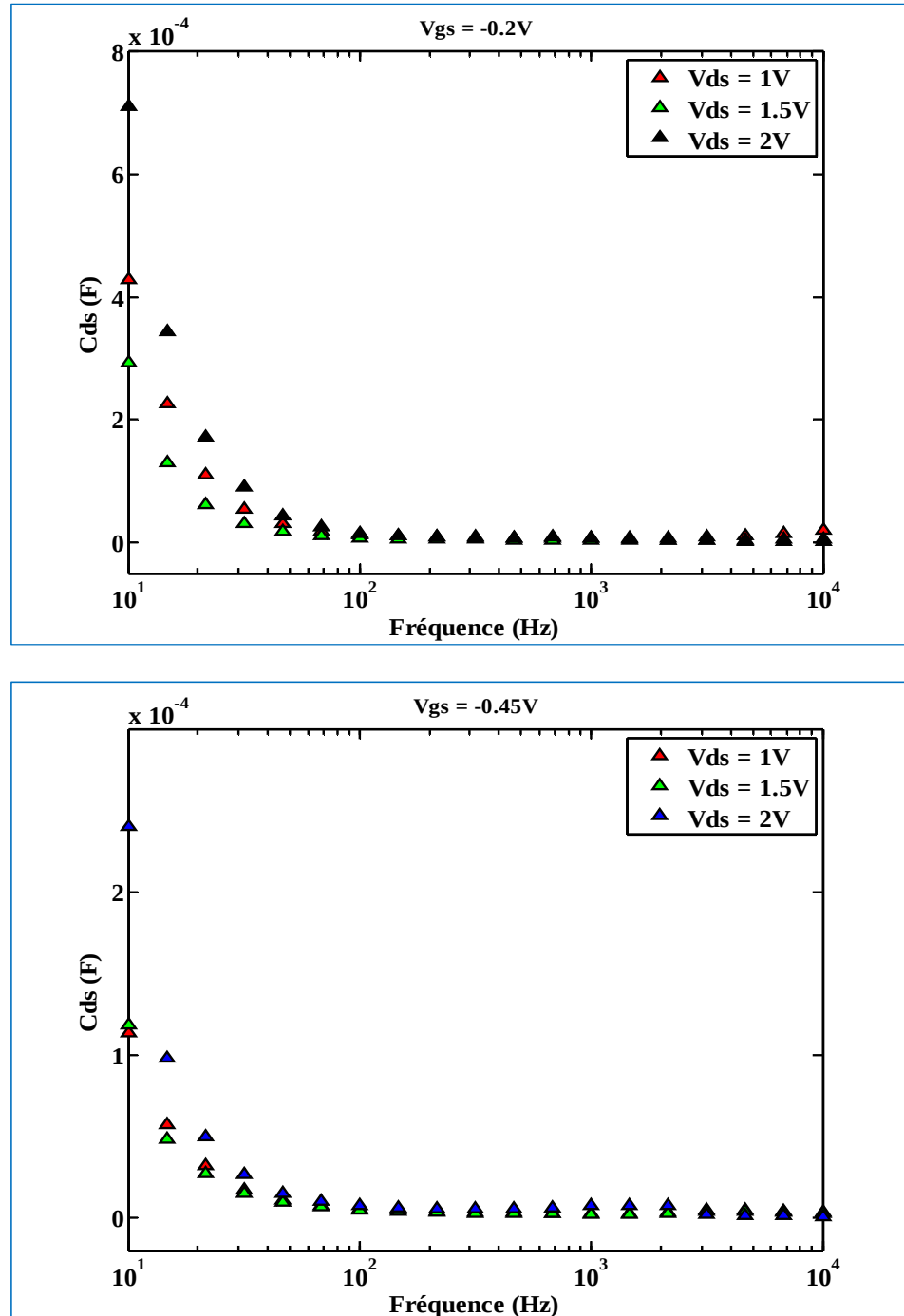
Fig. III. 8: Variation de la capacité de sortie en fonction de la fréquence, résultats expérimentaux à différents points de polarisation de drain:
