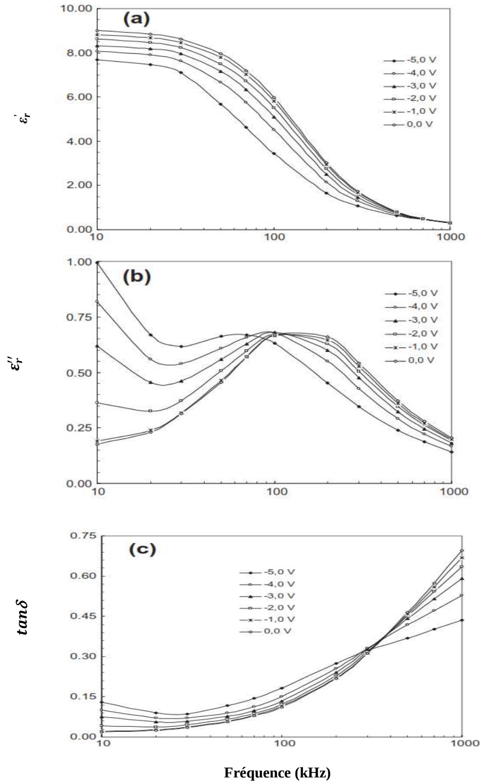
Fig. II. 4: Dépendance en fréquence de la partie réelle de la permittivité (a), la partie imaginaire (b), et la tangente de perte (c), d'une hétérostructure (\text{Ni/Au})/\text{GaN}/\text{Al}_{0.3}\text{Ga}_{0.7}\text{N} à différentes tensions de polarisation et à température ambiante [44].
