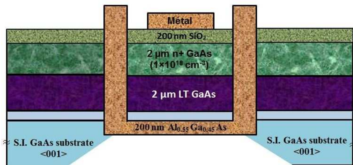
Fig. II. 7: Représentation schématique de la structure multicouche à base de GaAs [47].
