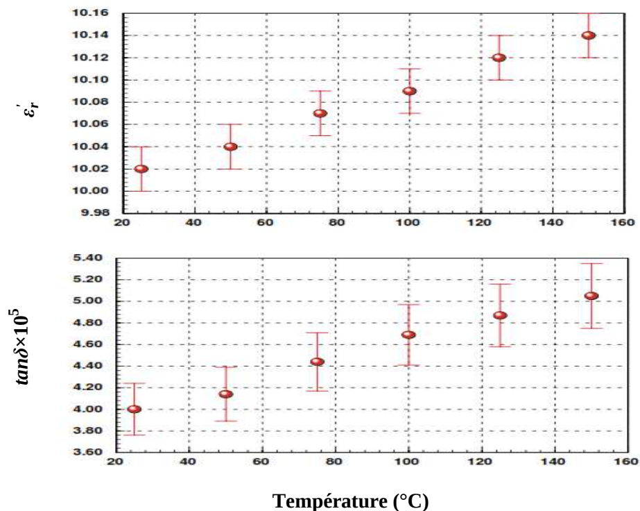
Fig. I. 2: Variation de la partie réelle de la permittivité et la tangente de perte de l'alumine en fonction de la température ( f = 7.53 GHz) [21].
