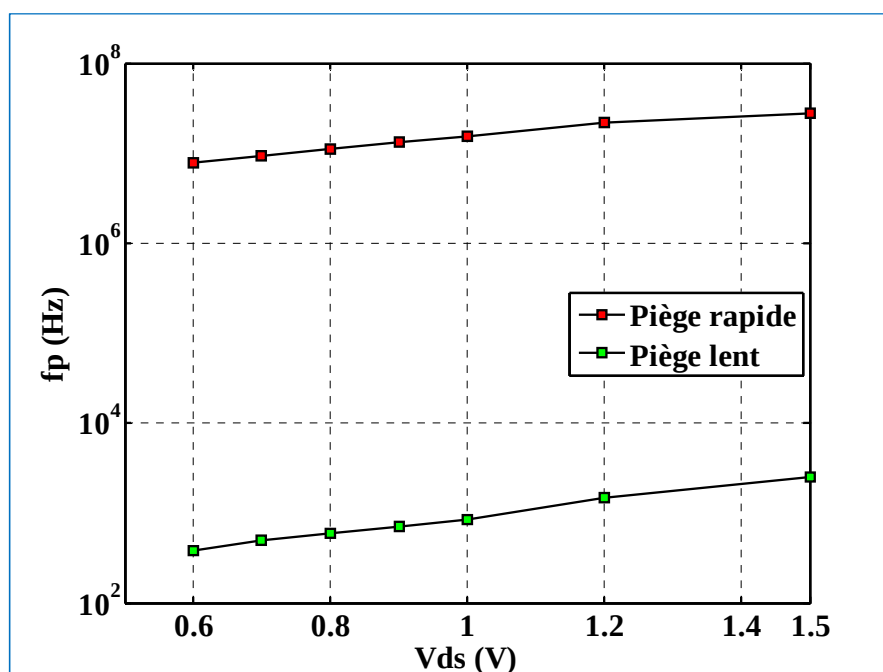
Fig. IV. 31: Variation de la fréquence du pic en fonction de la tension V_{ds} , pour les deux types de pièges.
