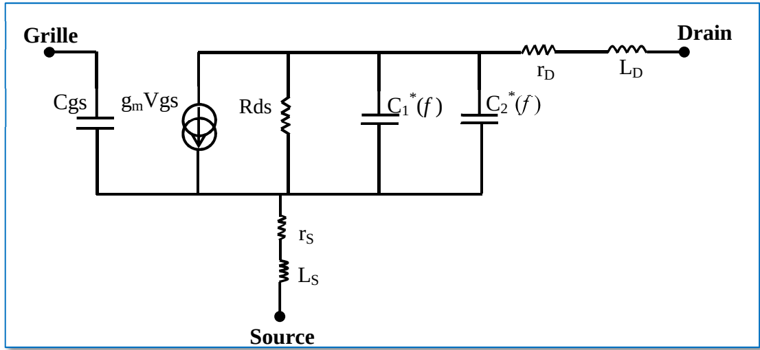
Fig. III. 11: Circuit équivalent de MESFET incluant la capacité de l'interface.
