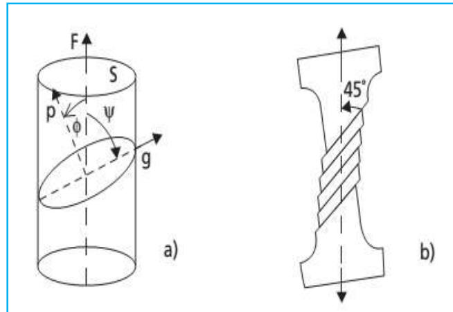
Figure I.11 : Glissement des plans atomiques denses dans un monocristal en traction. [16]
