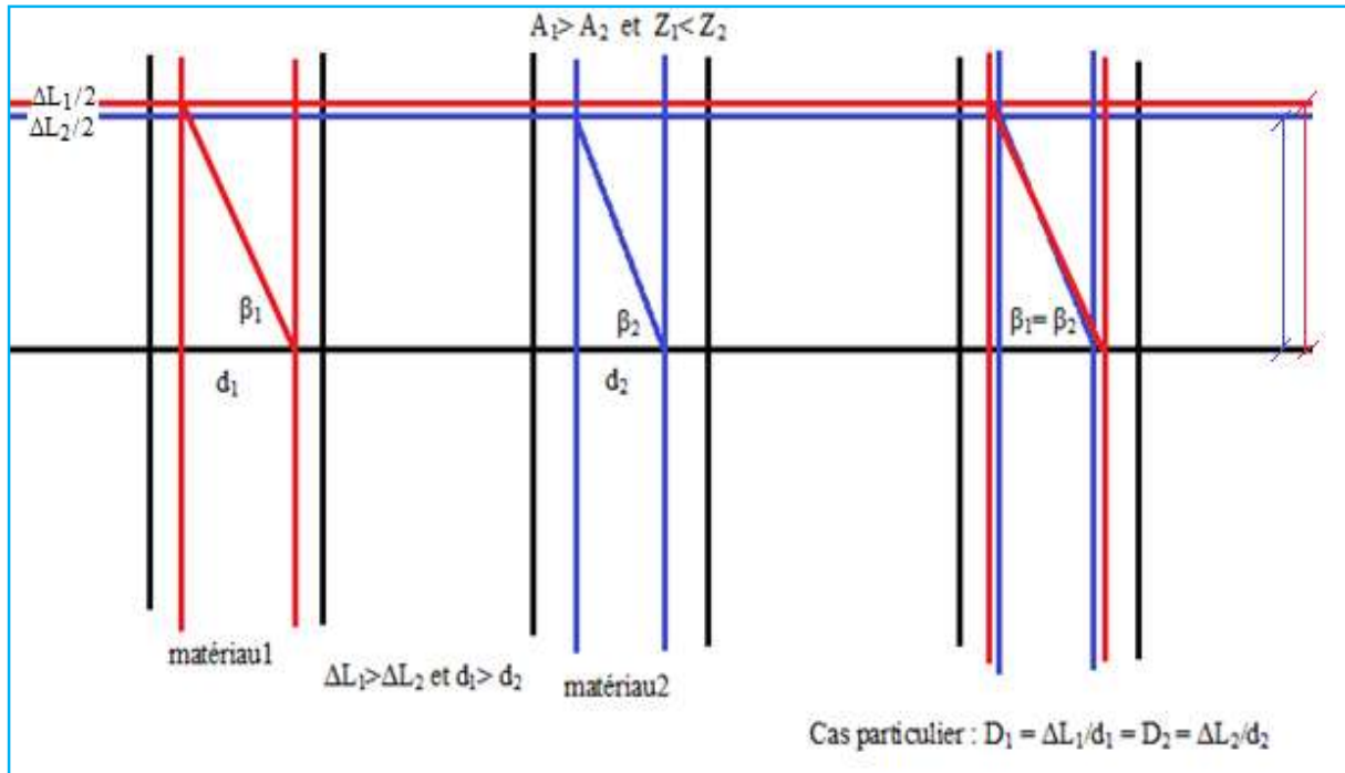
Figure III.30 représentation géométrique de l'approche D_1 de 02 matériaux 1et 2 d'allongement A_1 > A_2 et de striction Z_1 < Z_2 avec superposition des triangles 1et 2. D'après (figure III.30) on voit que le triangle de ductilité du matériau 1 a un angle de ductilité \beta_1 = \beta_2 du triangle de ductilité du matériau 2 ce qui implique que tg\beta_2 = tg\beta_1 .
