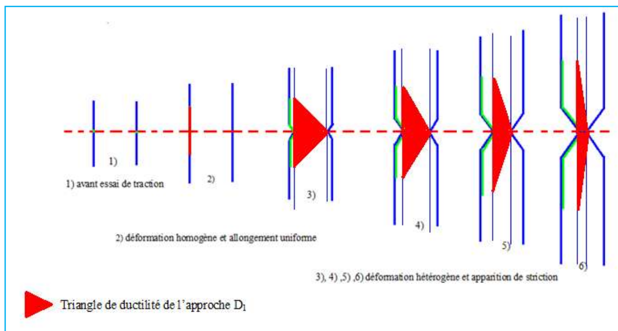
Figure II.9 : évolution géométrique du paramètre d’approche D_1 sur une éprouvette en traction.
