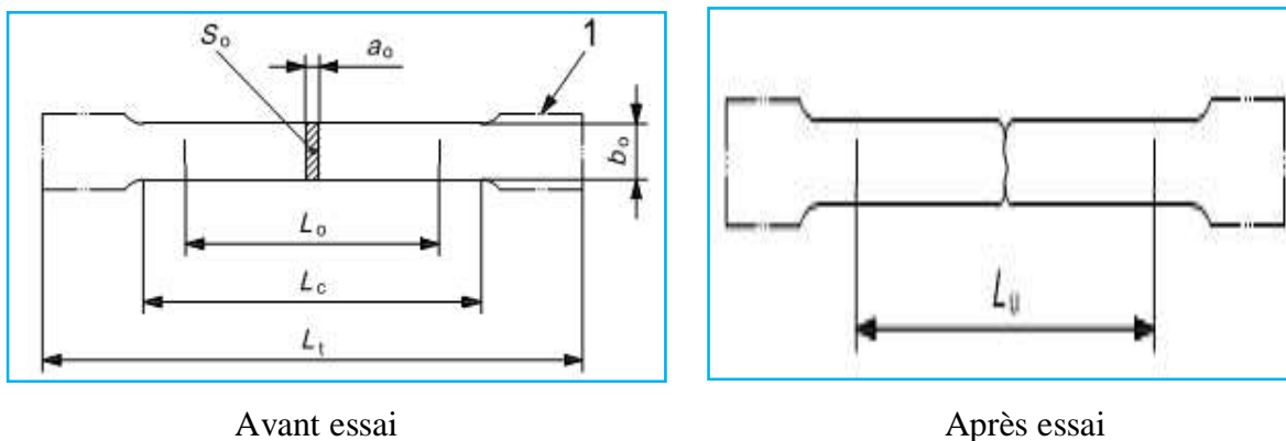
Figure I.29 : Forme et dimensions normalisée d'une éprouvette plate de traction avant et après essai. [45]
