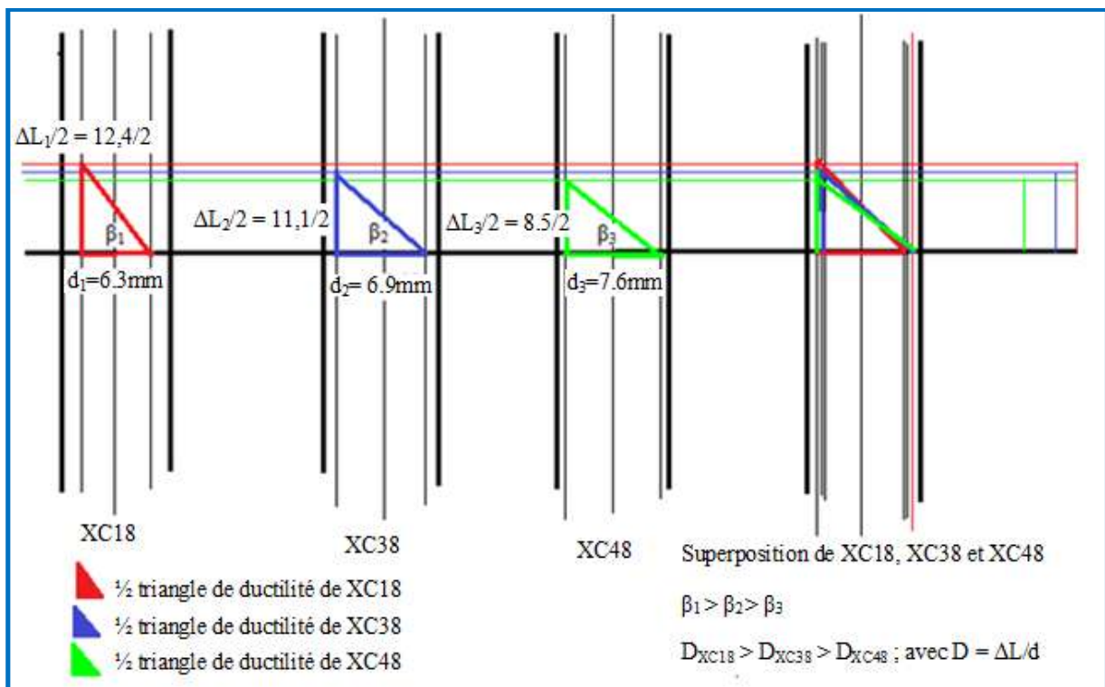
Figure III.26 : représentation géométrique de l'approche D_1 des aciers XC18, XC38 et XC48
