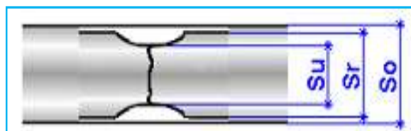
Figure I.33 : section éprouvette avant et après rupture
