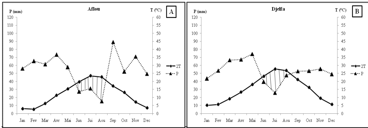
Figure 2. Diagramme Ombrothermique de Gaussen (2005-2014)
