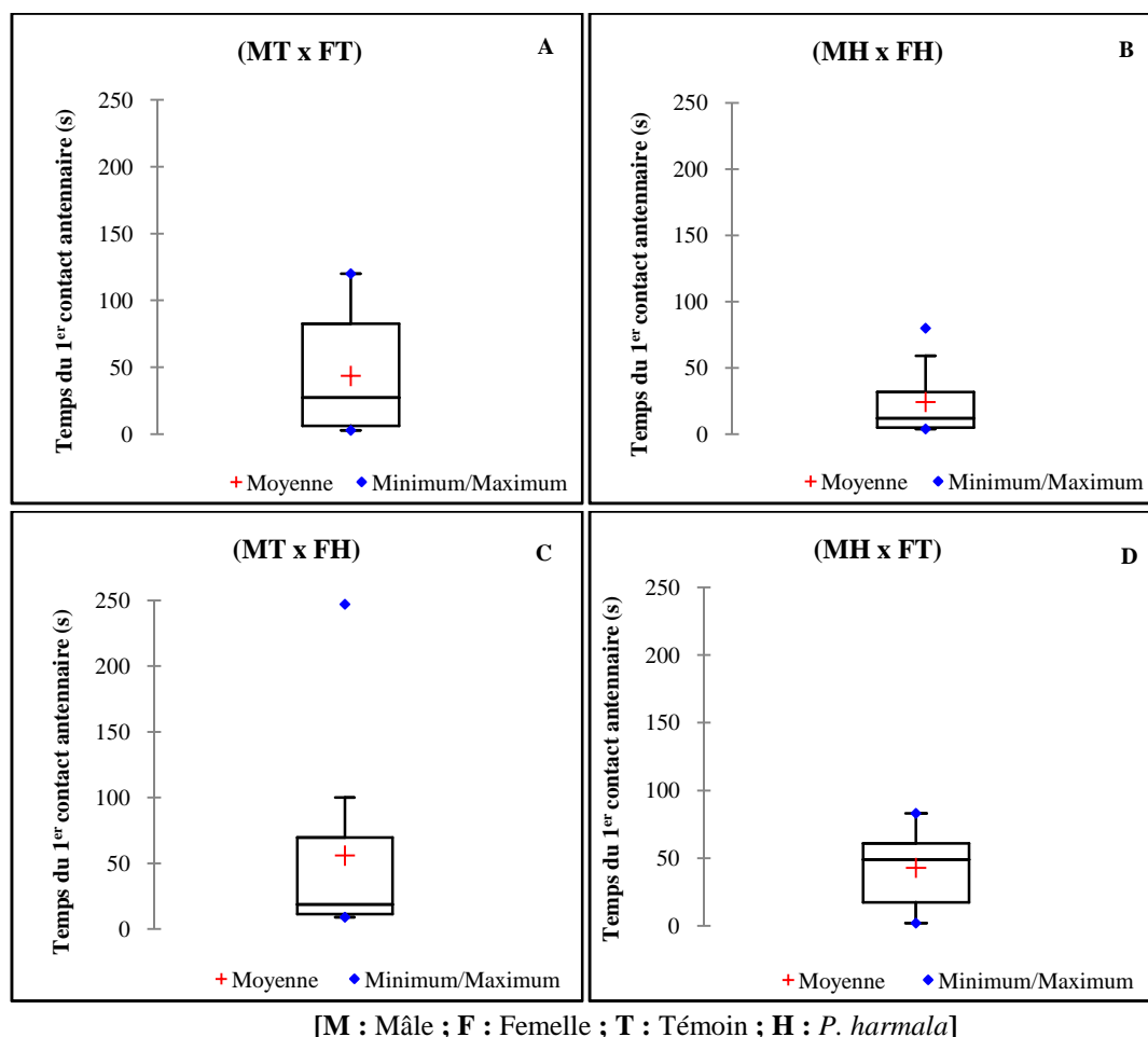
Figure 40. Effet de l'extrait aqueux des fleurs de P. harmala (700 \mu\text{g/ml} ) sur le temps (secondes) du premier contact antennaire
