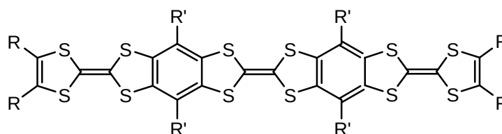
tri-TTF condensé
