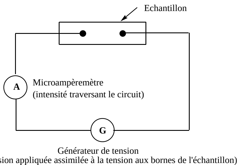
Figure 26 : montage de la mesure à deux contacts de la conductivité d'un sel.
