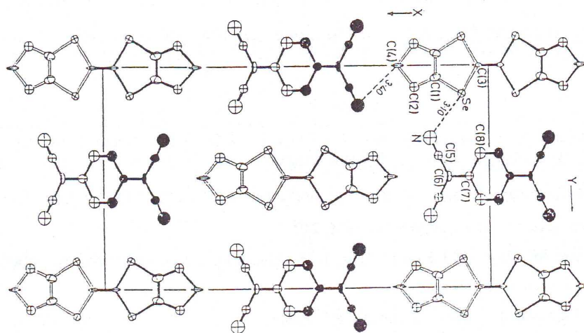
Figure 5 : Structure cristalline de type alterné du HMTSF-TCNQ.
