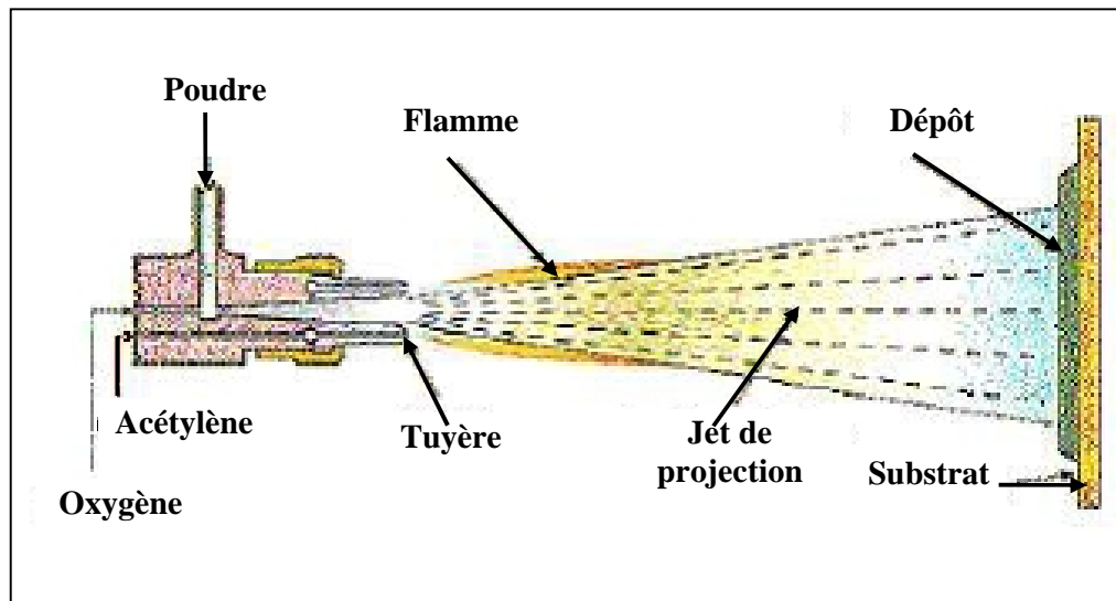
Figure I.2: Schéma du principe d'un pistolet flamme poudre [9]
