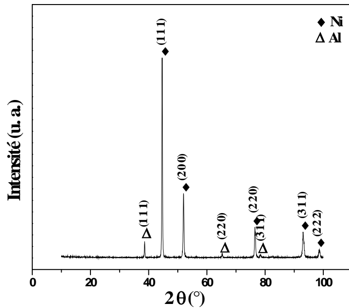
Figure III.7 : Spectre des rayons X de la poudre de Ni-5wt%Al
