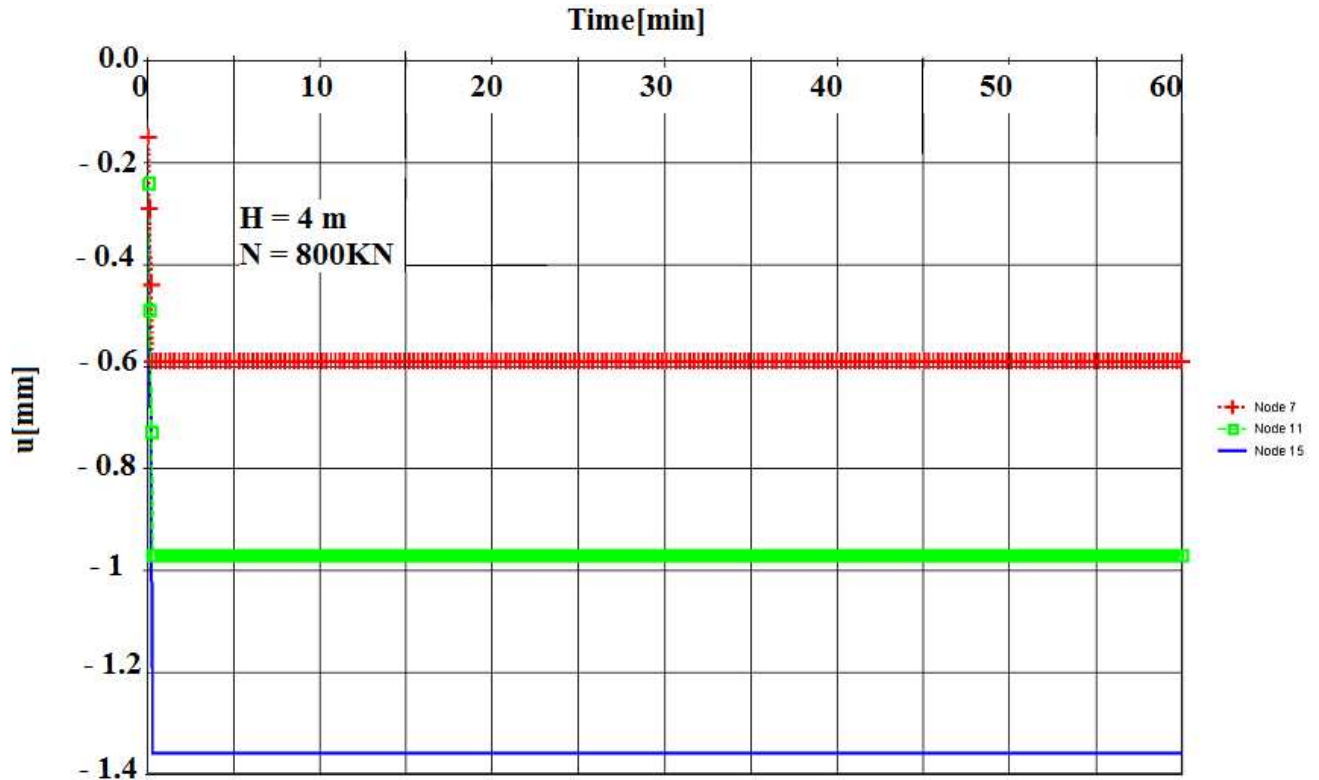
Figure 2.38: Déplacements verticaux à froid de la colonne D_6
