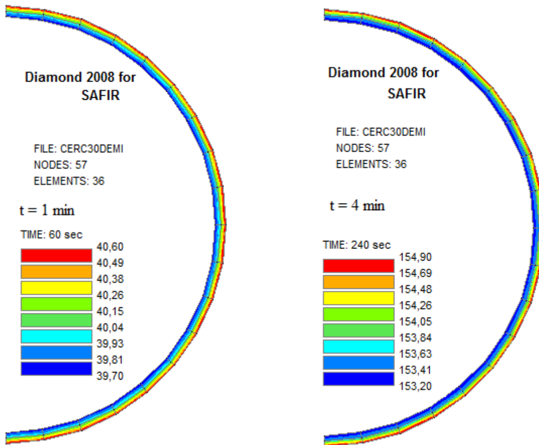
Figure 3.9- Température du poteau circulaire après 60s et 240s
