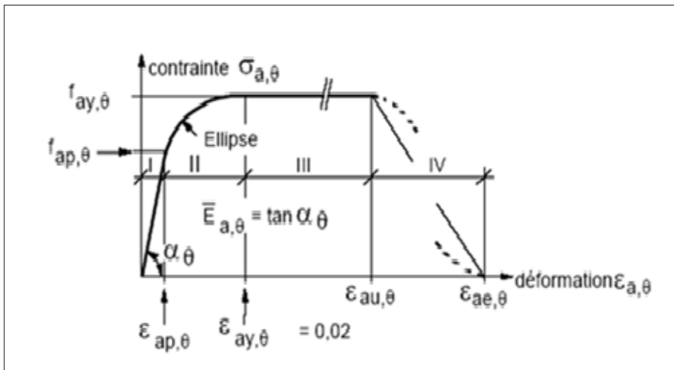
Figure 1.5- Modèle de la relation contrainte – déformation acier aux températures élevées
