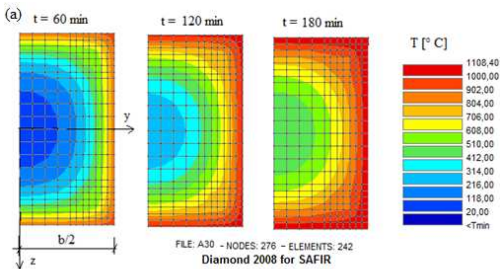
Figure 2.21 Calcul isothermal aux temps : t = 60, 120, 180 min
