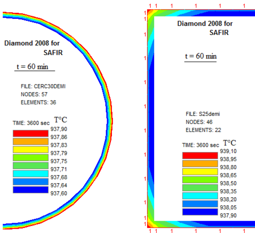
Figure 3.15- Température des poteaux en carré et circulaire après 60 min
