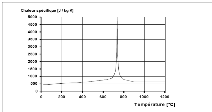
Figure 1.1 Chaleur spécifique de l'acier [ENV, 93]
