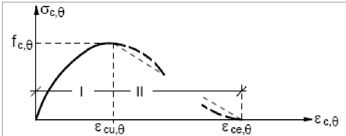
Figure 1.7 : Modèle mathématique à température élevée des relations contrainte- déformation du béton en compression proposée par L'Euro code 4[ENV, 94]
