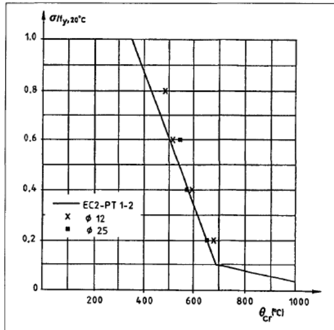
Figure 1.20 – Essais transitoires. Variation du niveau de contrainte en fonction de la température critique
