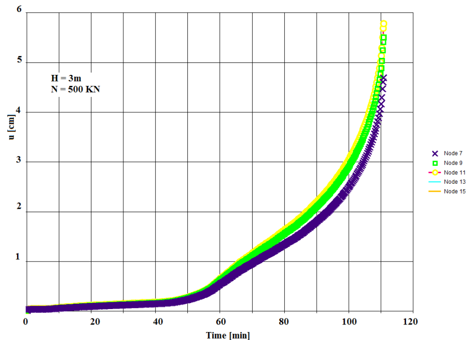
Figure 2.32 Déplacement latéral pour cinq nœuds de la colonne B 3
