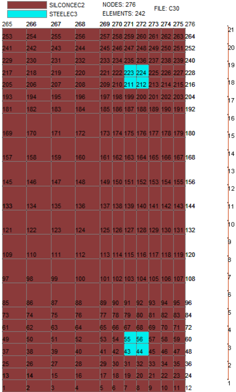
Figure 2.14 Numérotation des nœuds de la demi section
