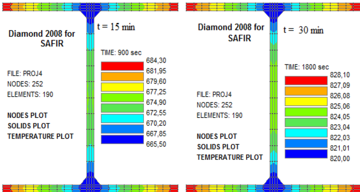
Figure 3.14 - Température du poteau en I après 15 min et 30 min
