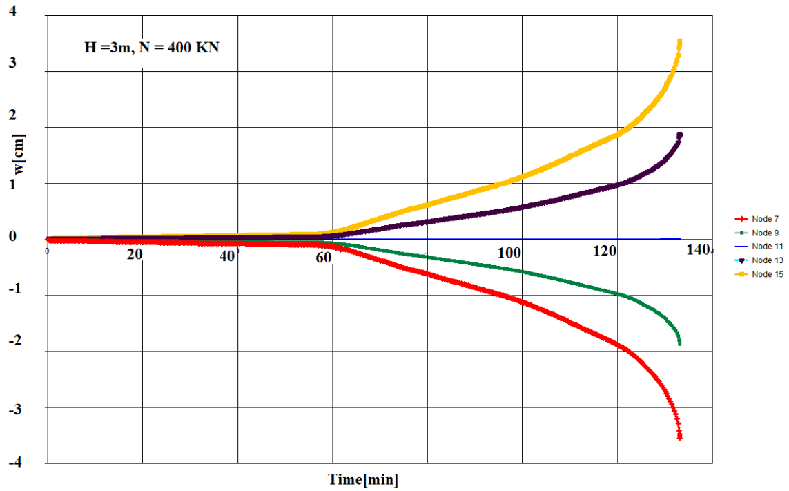
Figure 3 : Rotation des nœuds de la colonne B 2
