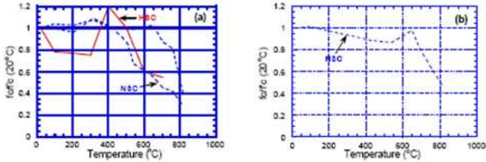
Figure 1.11 Résistance de compression du béton - température pour (a) NWA et (b) LWA (stressed tests)
