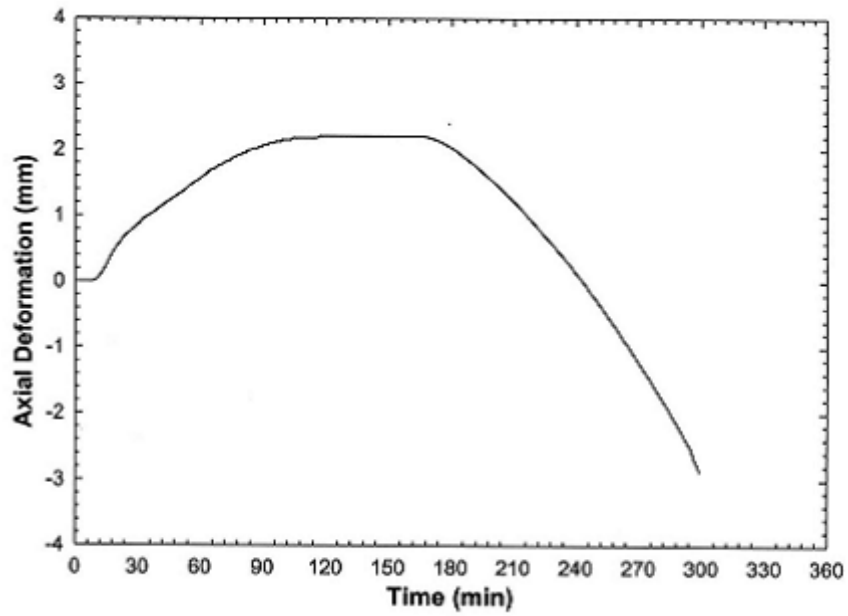
Figure. 2.12- Déformation axiale en fonction du temps dans la colonne HS2-1
