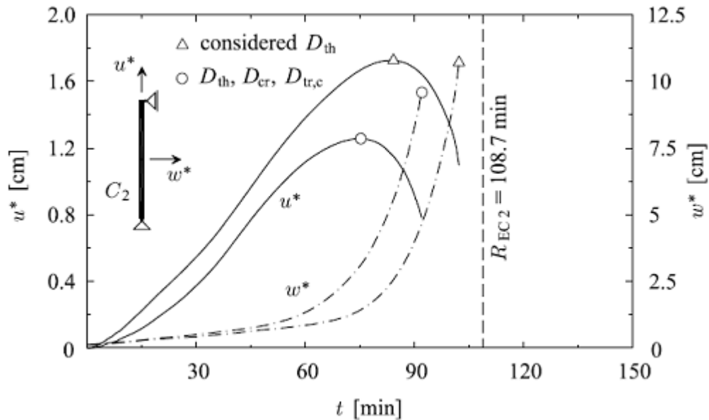
Figure 2.10 : Variation du déplacement axial et latéral de la colonne C_2 (charge excentrée). (Triangles) seulement la déformation thermique ( D_{th} ) est prise en compte. (cercles) déformation due au fluage ( D_{th}, D_{cr}, D_{tr,c} ) non négligée.
