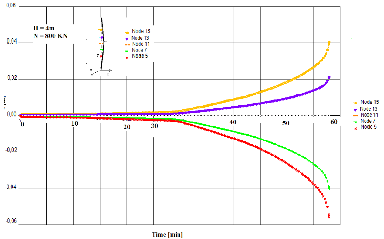
Figure 2.29 : Rotations des nœuds 5, 7, 11, 13, 15 de la colonne D_6
