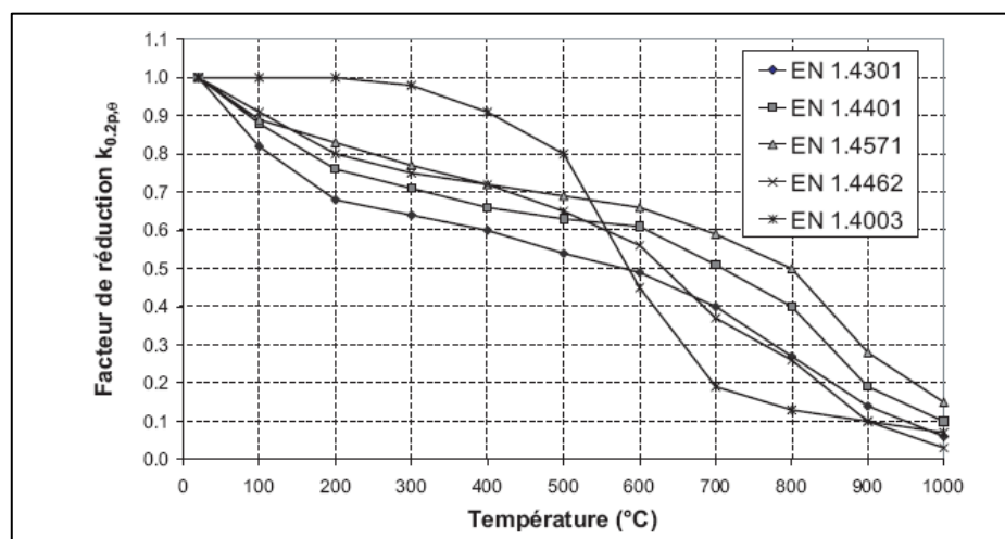
Figure 1.7 – Évolution du facteur de réduction de la limite d'élasticité à 0,2 % de déformation plastique des aciers inoxydables en fonction de la température [ZHA, 02]
