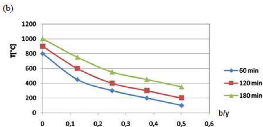
Figure 2.22 Evolution de la température dans la section de béton
