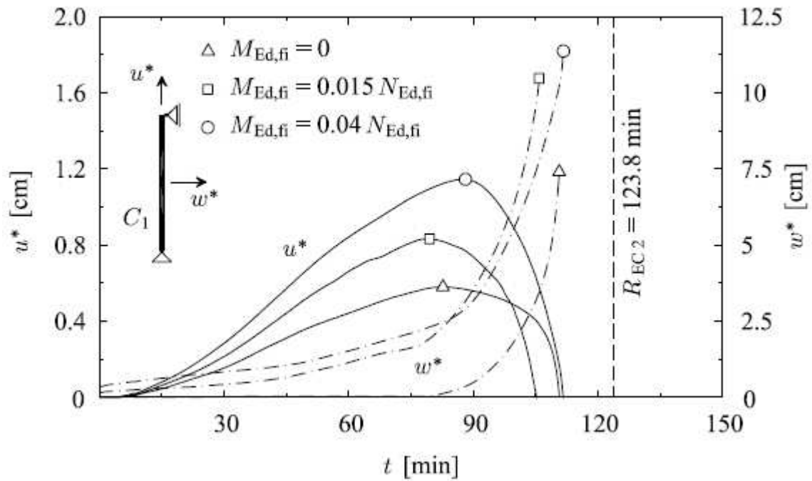
Figure 2.11. Variation du déplacement axial et latéral de la colonne C_1 . Déformation due au fluage et à la charge non négligées.
