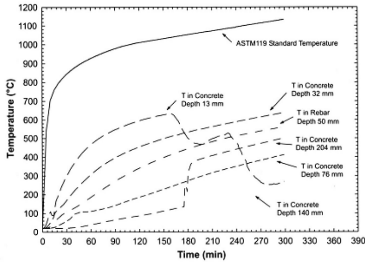
Figure 2.2- Courbes des températures en fonction du temps dans la colonne HS2-1
