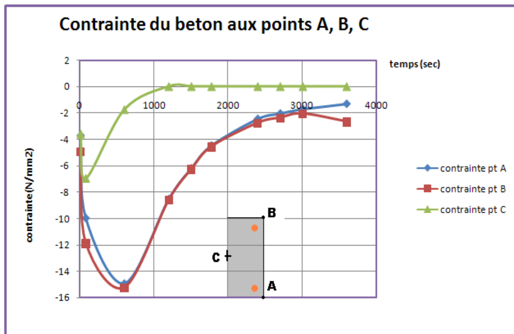
Figure 2.27: Variation des contraintes du béton
