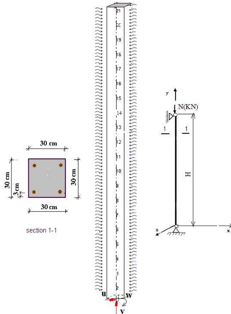
Figure 2.24: Schématisation des colonnes considérées
