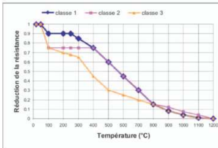
Fig. 1.9- Diminution de la résistance à la compression des bétons haute résistance. Les classes sont fonction de la résistance [DEN, 07]
