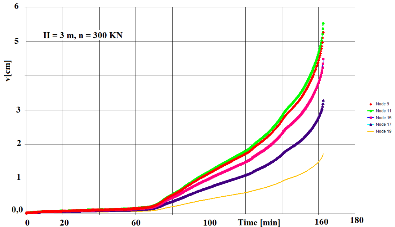
Figure 2.37 Déplacement latéral pour cinq nœuds de la colonne B 1
