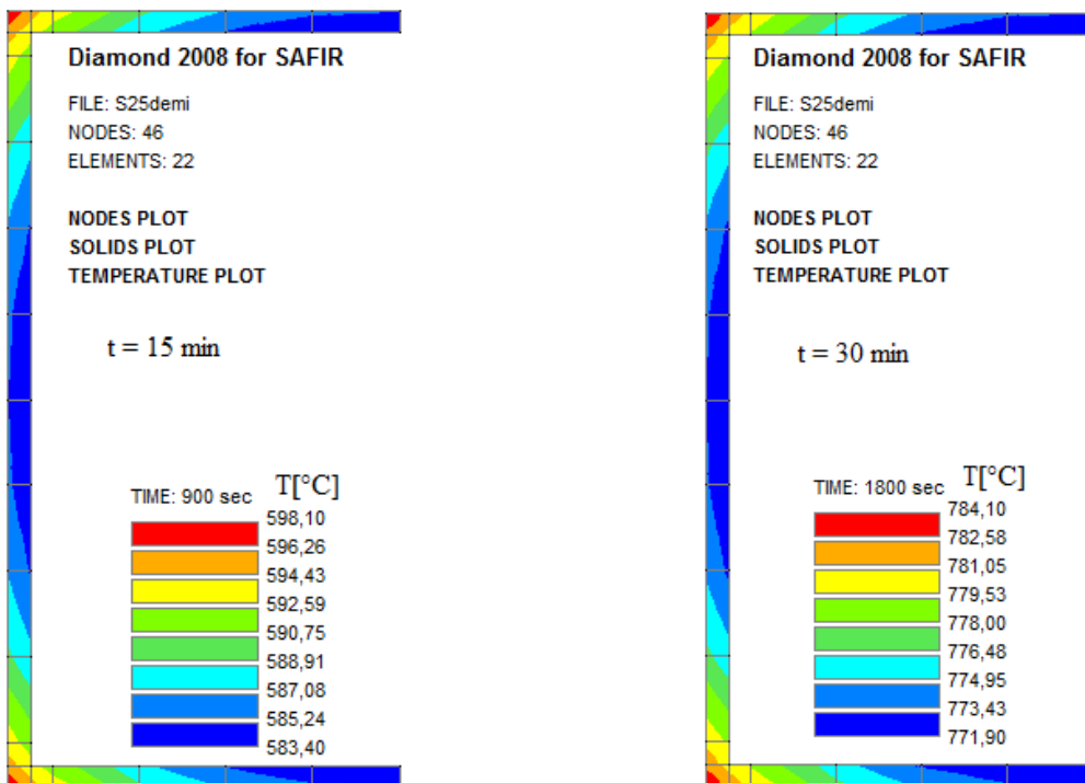
Figure 3.12- Température du poteau carré après 15min et 30 min
