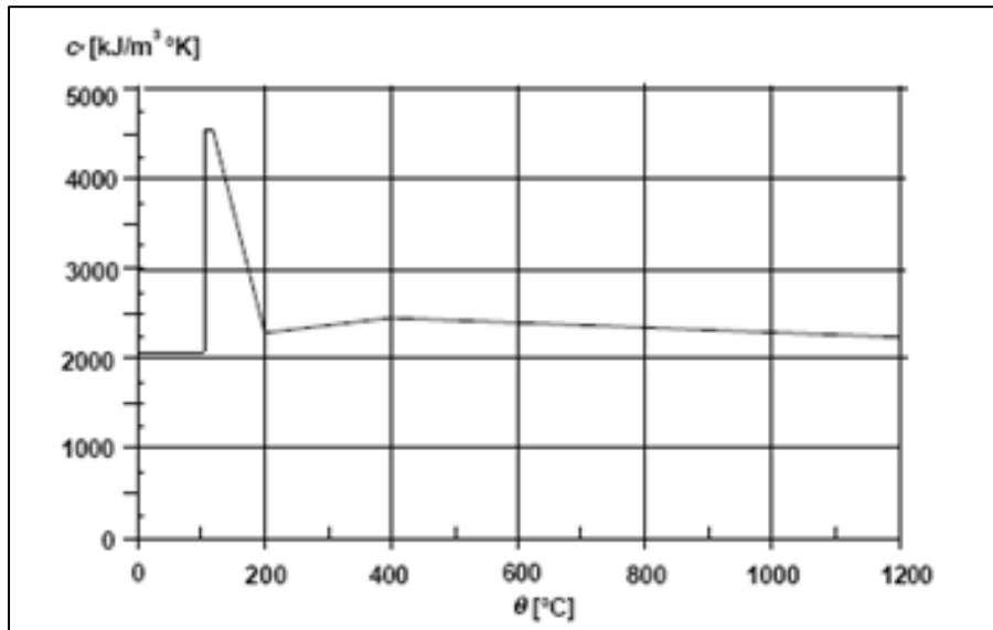
Figure 1.5 : Chaleur spécifique volumique
