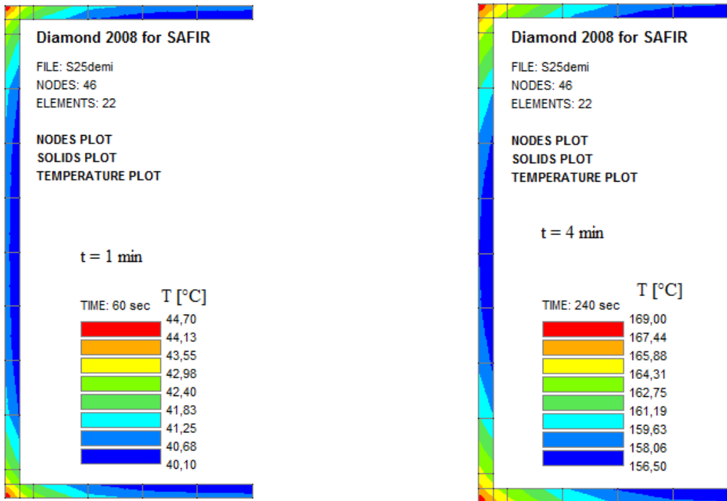
Figure 3.11- Température du poteau carré après 60s et 240s
