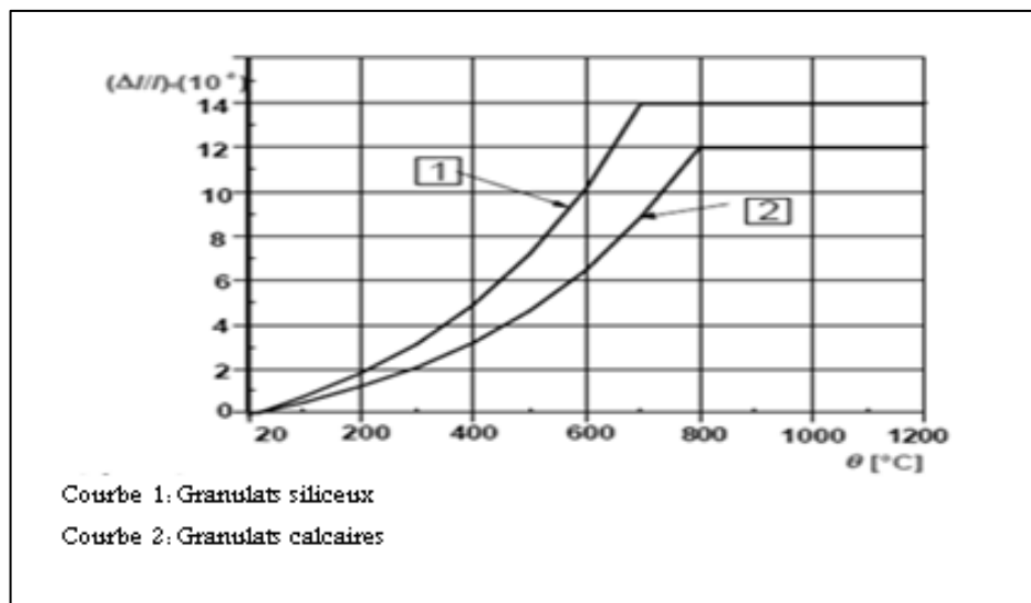
Figure 1.3 : dilatation thermique totale du béton.
