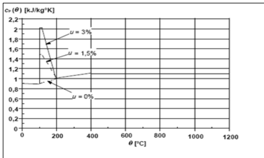
Figure 1.4 : Chaleur spécifique
