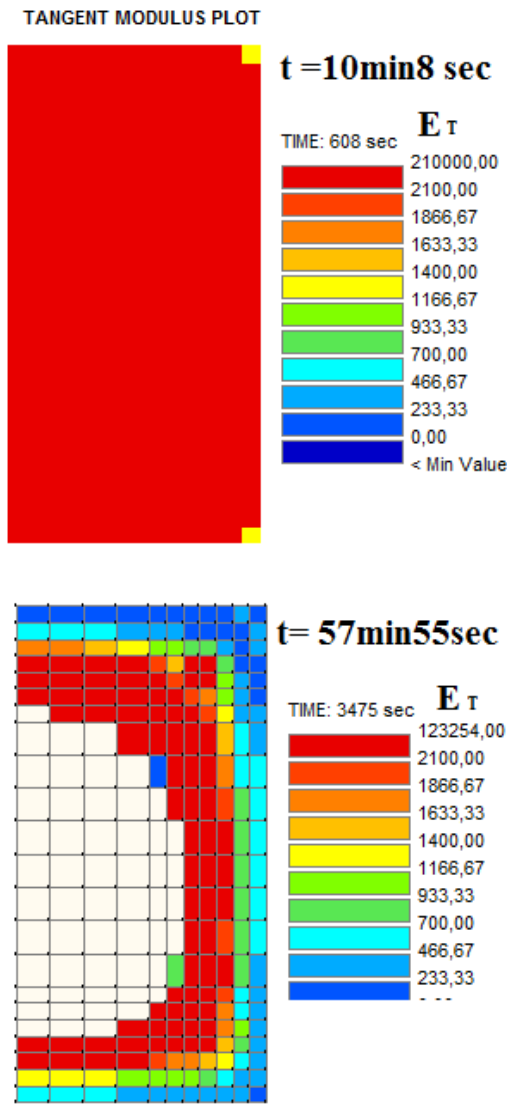
Figure2.31 : Module tangent de la colonne D 6
