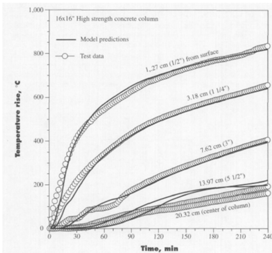
Figure 2.6 Validation de l'évolution de la température pour une colonne en béton à haute résistance HSC avec agrégats de carbone le long d'une ligne normale à l'axe centrale jusqu'à la surface [AHM, 99]
