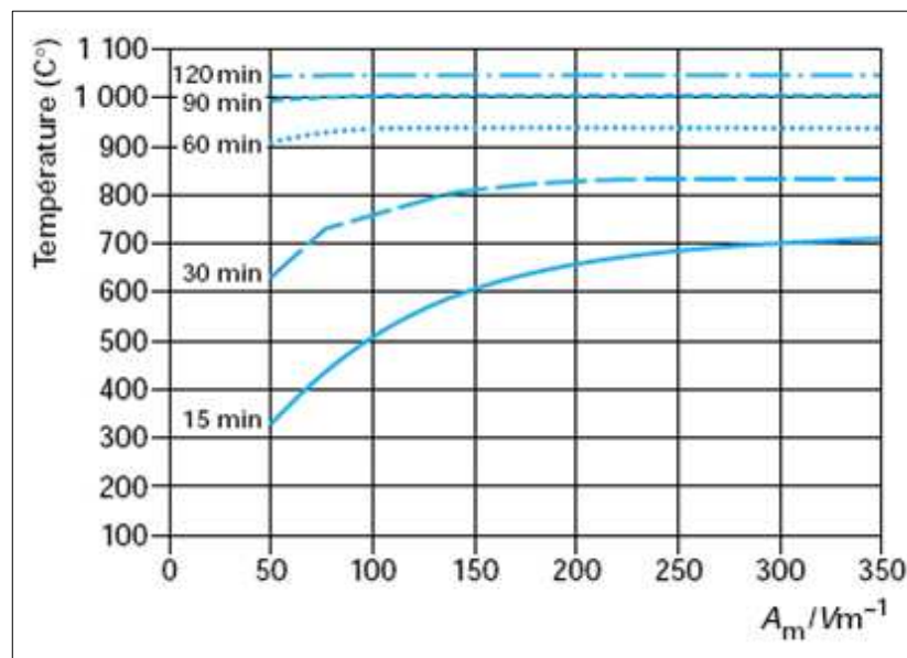
Figure 2.1 – Température de profilés en acier en fonction de leur facteur de massivité (en m^{-1} ) et de la durée d'échauffement sous incendie conventionnel
