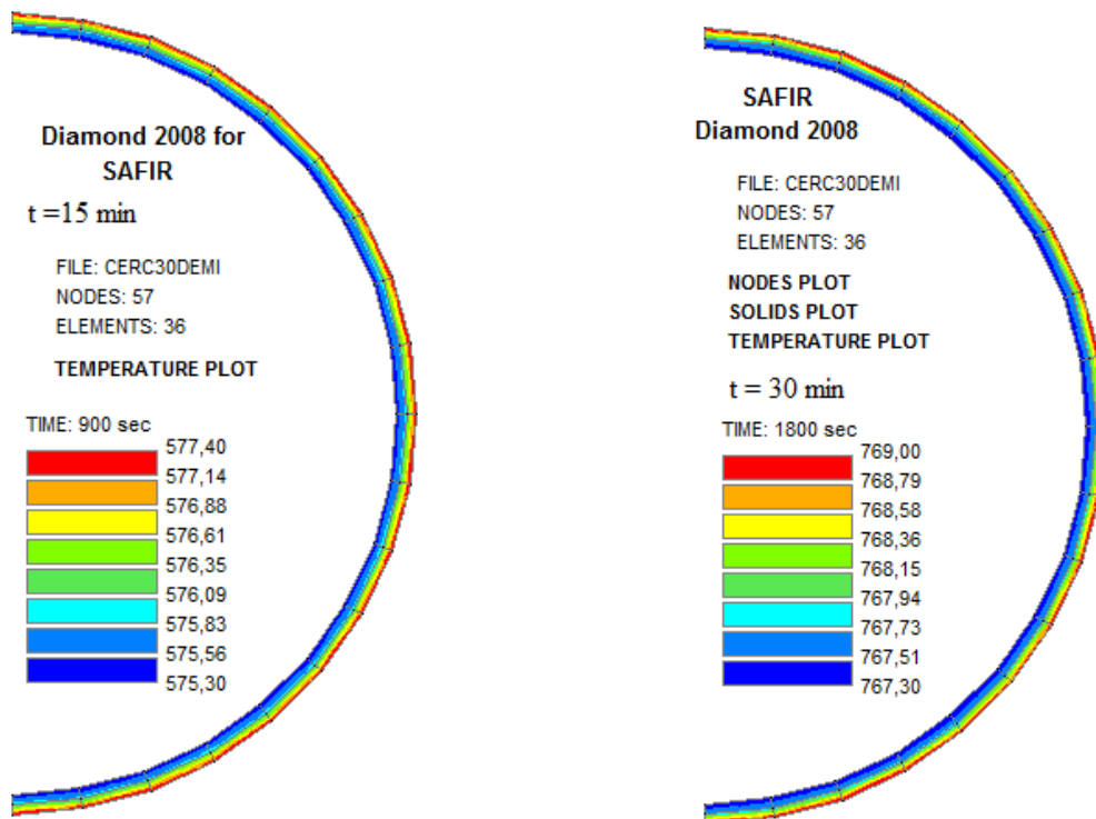
Figure 3.10- Température du poteau circulaire après 15min et 30 min
