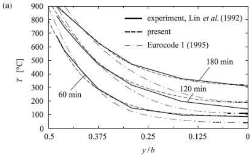
Figure.2.7 Comparaison entre les températures calculées, de colonnes en béton armé, avec des résultats expérimentaux et avec l’Eurocode.
