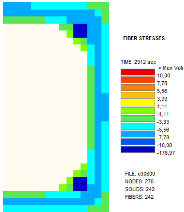
Figure 5 : Contraintes à t = 48min32sec
