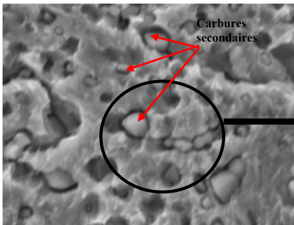
Figure 3.71. : Micrographie MEB (X15000) d'une plage de matrice de la fonte traitée à 0.5%(Mn+Ti)
