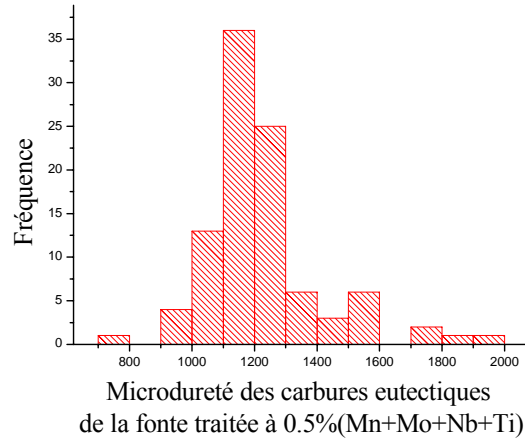
Figure 3.41. : Distribution de la microdureté des carbures eutectiques de la fonte traitée à 0.5%(Mn+Mo+Nb+Ti)
