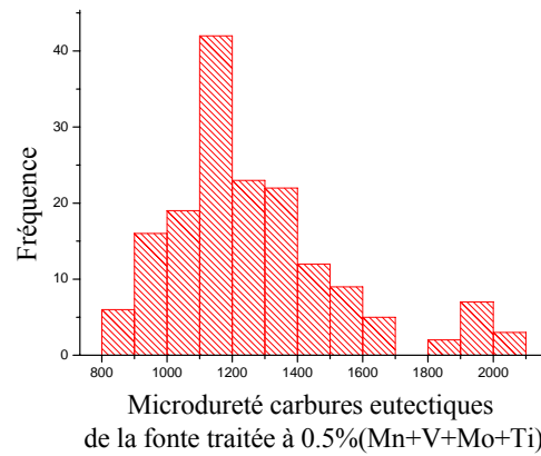
Figure 3.43. : Distribution de la microdureté des carbures eutectiques de la fonte traitée à 0.5%(Mn+Mo+V+Ti)
