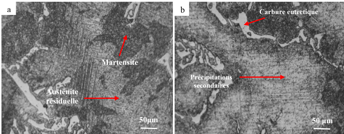
Figure 3.8. : Micrographie de la fonte traitée à 0.5% (Mn+Mo)
