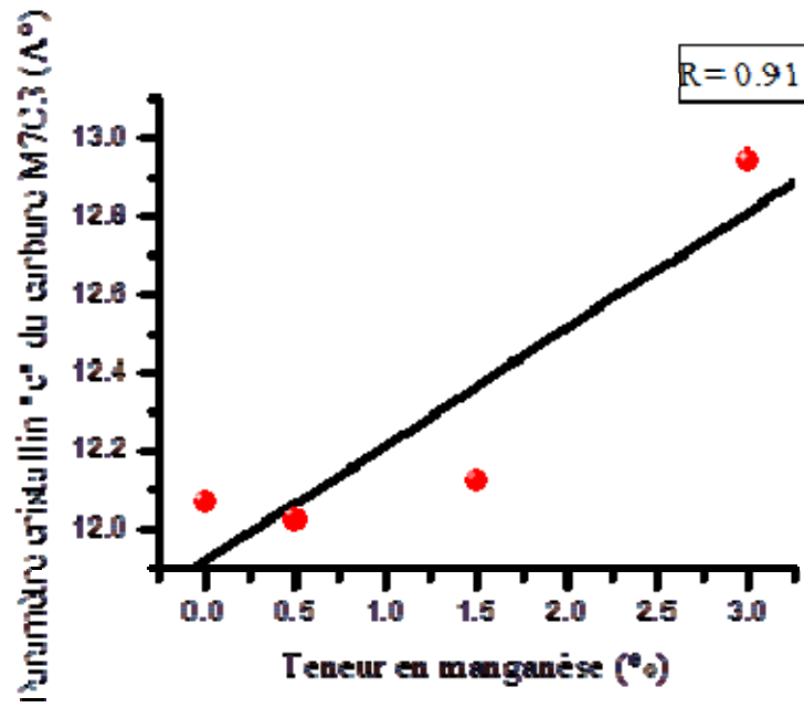
Figure 3.55. : Variation du paramètre cristallin «c» du carbure M_7C_3 orthorhombique
