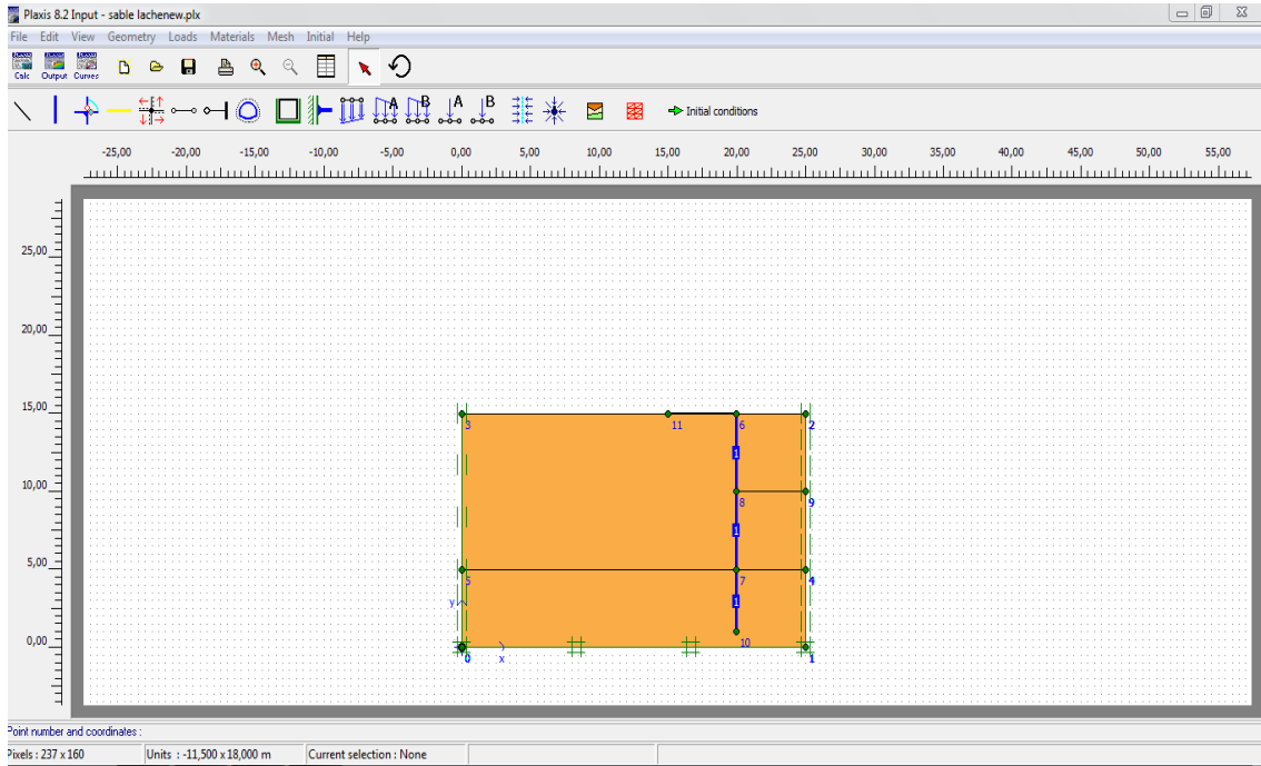
Figure III.16 . Définition de la géométrie d'un ancrage horizontal a la surface du sol (sable lâche)
