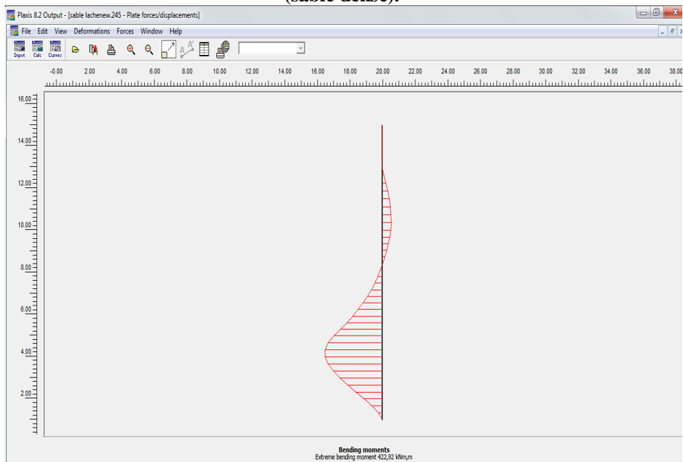
Figure III.43 . Moment fléchissant d'un ancrage situe a 3 m de profondeur (sable dense)
