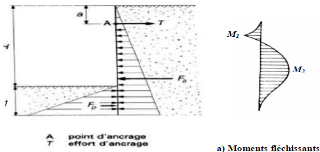
Figure II.7. Rideau ancré en tête simplement buté en pied.[6]
