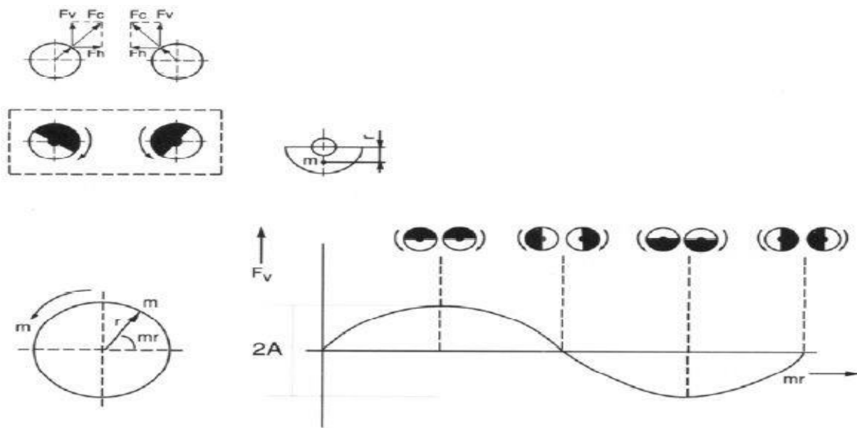
Figure I.23.Principe de fonctionnement d'un vibreur (brochure ICE).
