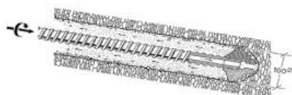
Trilame, vissable, pour sols cohérents, p.ex. dans les marnes
