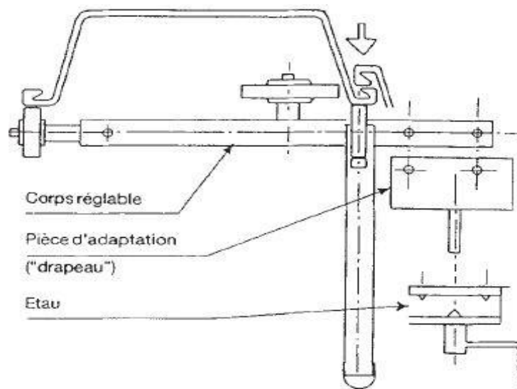
Figure I.24. Enclencheur automatique
