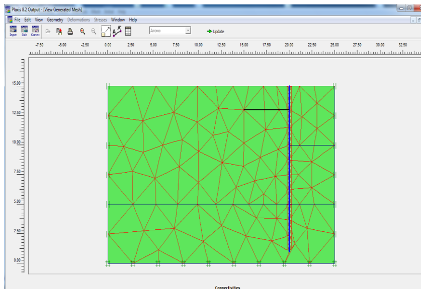
Figure III.39 . Maillage de l'excavation d'un ancrage situé a 2 m de profondeur (sable dense)
