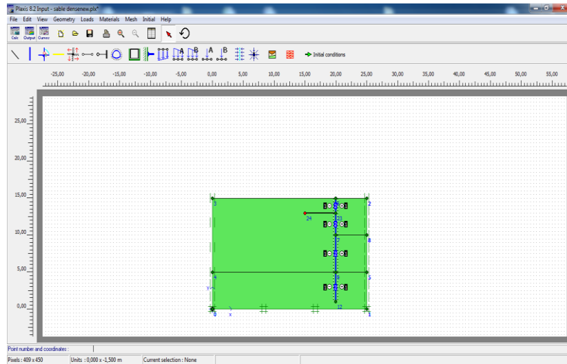
Figure III.38 . Définition de la géométrie d'un ancrage situé a 2m de profondeur (sable dense)
