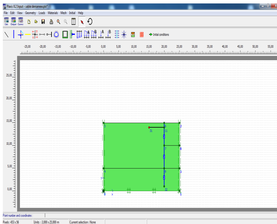
Figure III.35 . Définition de la géométrie d'un ancrage situe a 1m de profondeur (sable dense)
