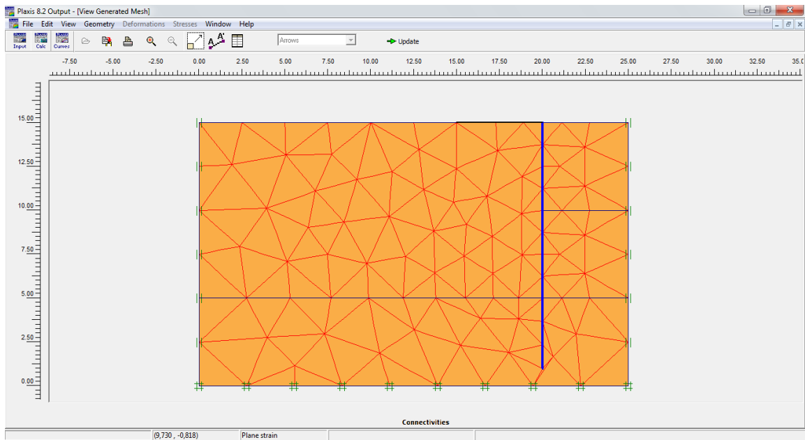
Figure III.17. Maillage de l'excavation d'un ancrage horizontal a la surface du sol (sable lâche)
