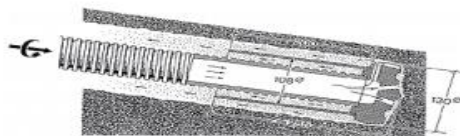
Pointe de sonnette, vissable, pour sols légers et compressibles, pour sols cohérents à haut niveau d'eau.
