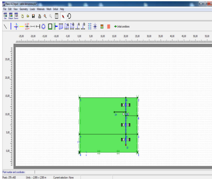
Figure III.45 . Définition de la géométrie d'un ancrage situe a 4 m de profondeur (sable dense).
