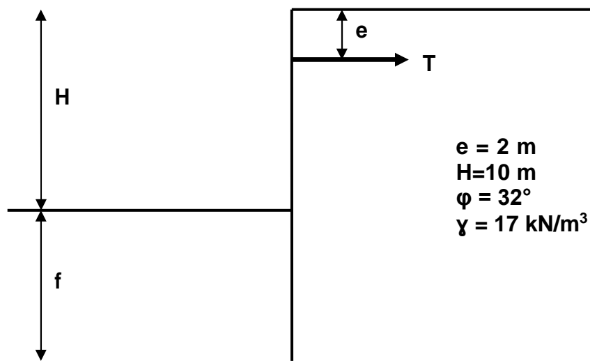
Figure III.04 palplanches avec ancrage
