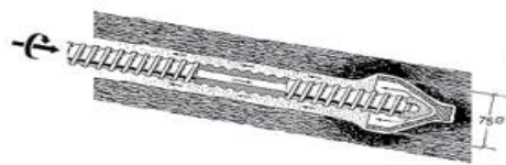
Pointe de sonnette, vissable, pour sols légers et compressibles, pour sols cohérents à haut niveau d'eau.
