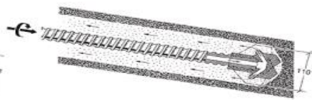
Taillant pour mono-jet clouté à 200 bars, vissable, avec 2 buses de 2,3 mm, dans la craie et l'argile
