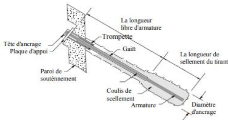
Figure I.28. Composants d'un tirant d'ancrage [11]
