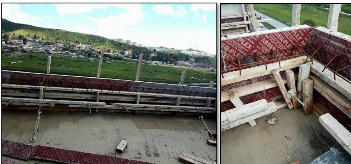
-Figure 7-10 : Coffrage et ferrailage du l'acrotère-
