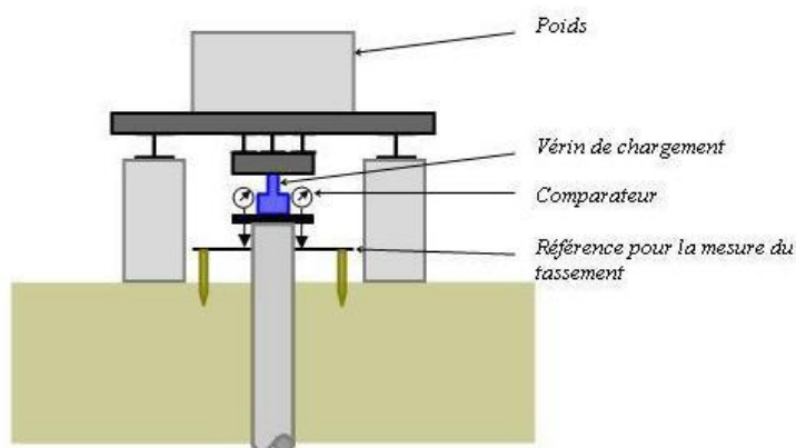
-Figure 5-6: Principe de l'essai de chargement-
