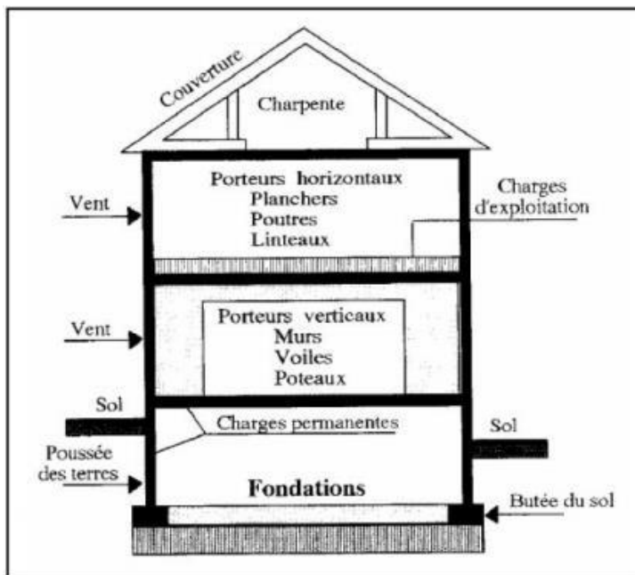
-Figure 5-2: Transmission des charges et surcharge au sol-
