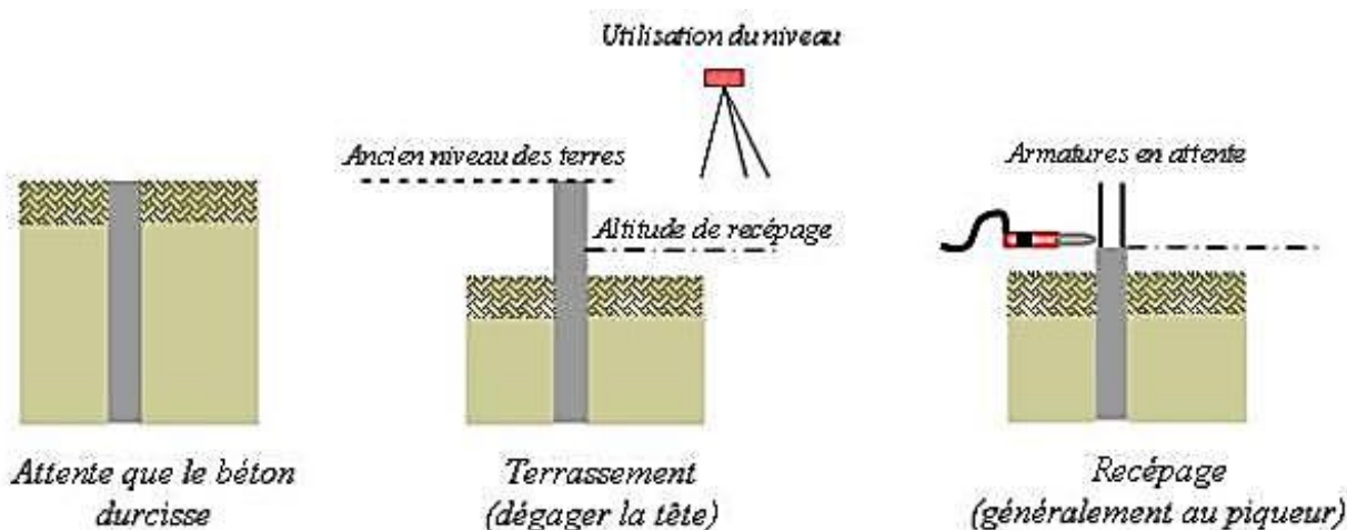
-Figure 5-30 : La technique du recépage par marteau piqueur -
