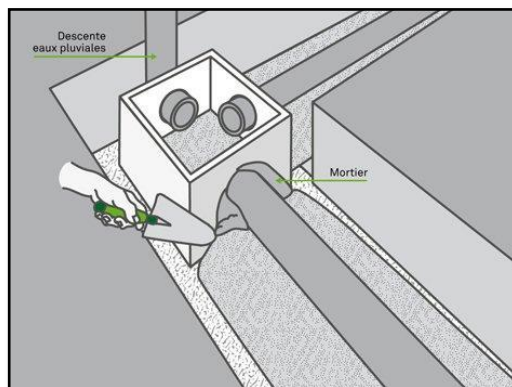
Figure 7-20 : L'étanchéité du raccordement
