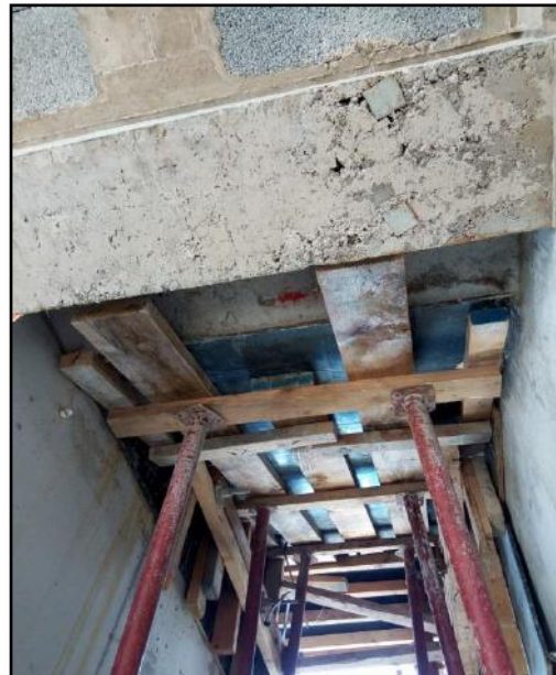
-Figure 7-6 : Coffrage d'escalier-
