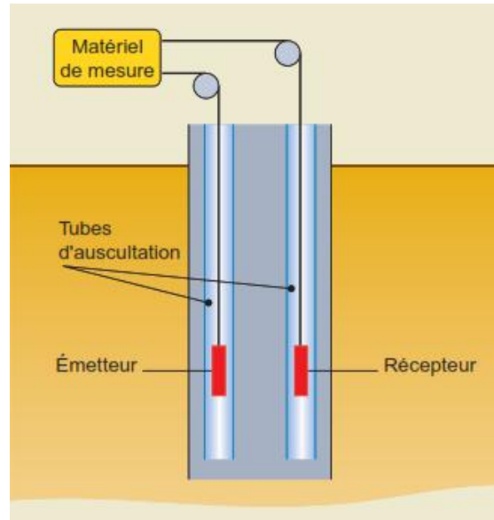
-Figure 5-10 : Schéma de principe-
