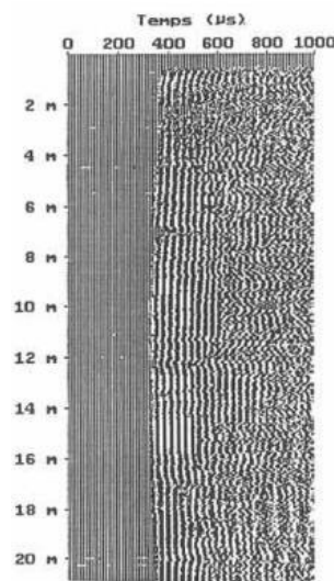
Figure 5-15 : Exemples d'enregistrement de l'amplitude et du temps sur un pieu
