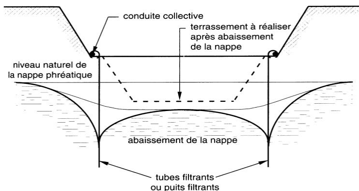
-Figure 5-22 : Rabattement de nappe-
