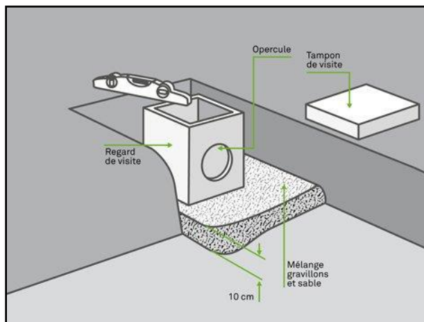
-Figure 7-19 : La pose des regards-
