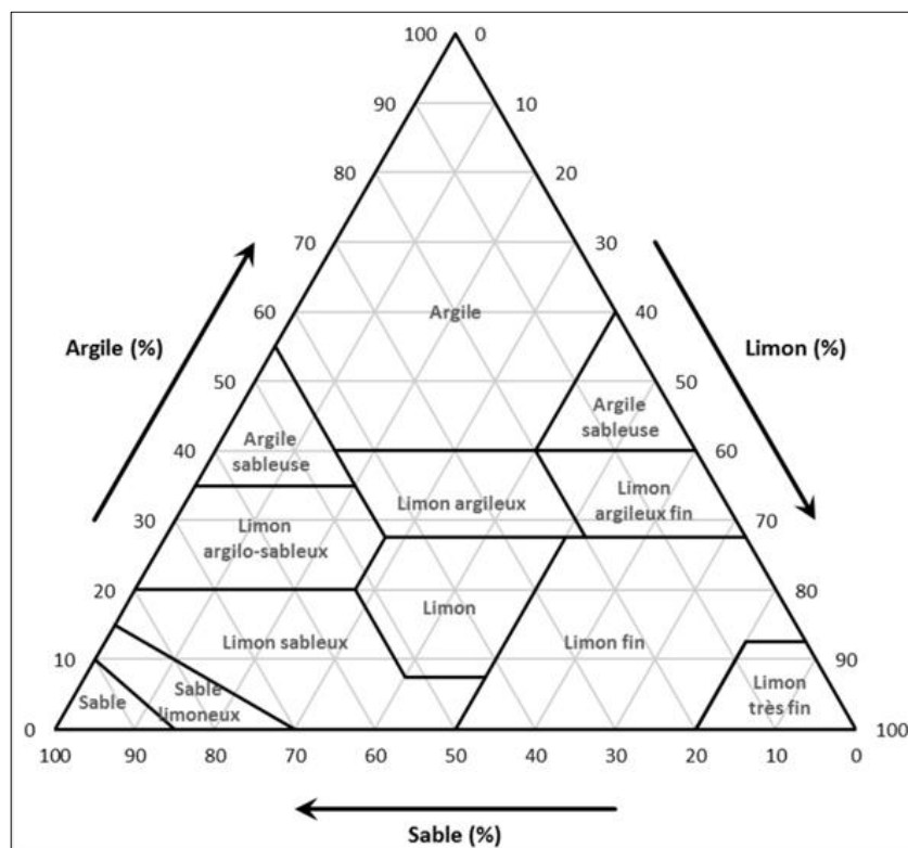
-Figure 4-1 : Texture du sol-
