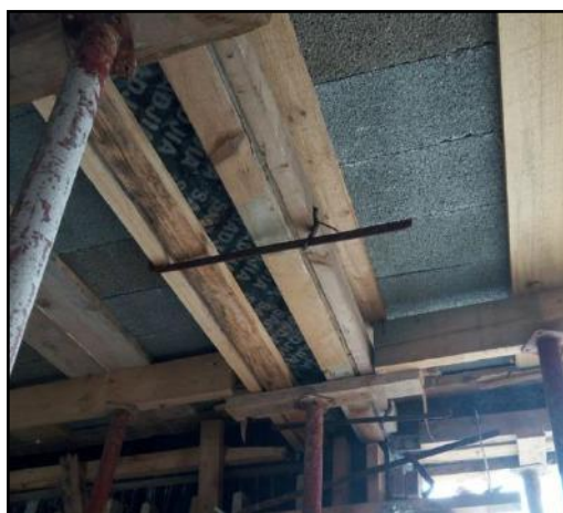
-Figure 7-3 : Coffrage du poutre-
