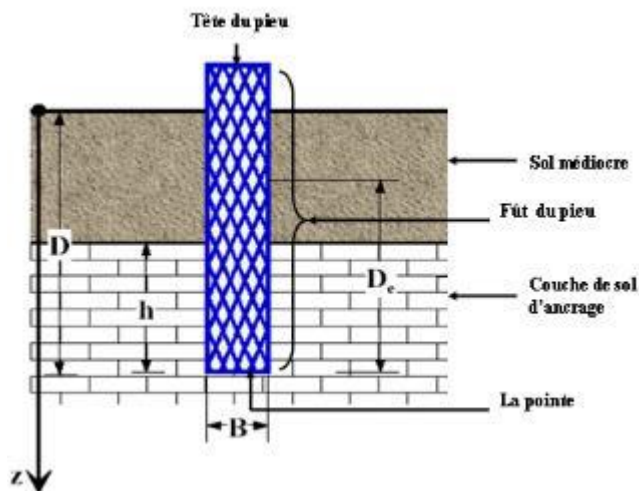
-Figure 5-5: Les parties principales d'un pieu-
