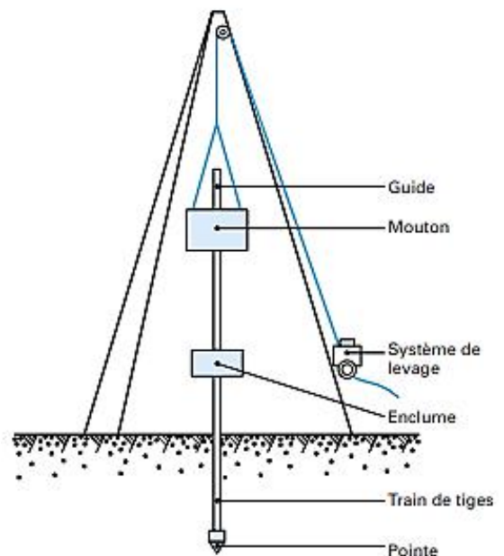
Figure 4-2 : Schéma de principe du pénétromètre dynamique
