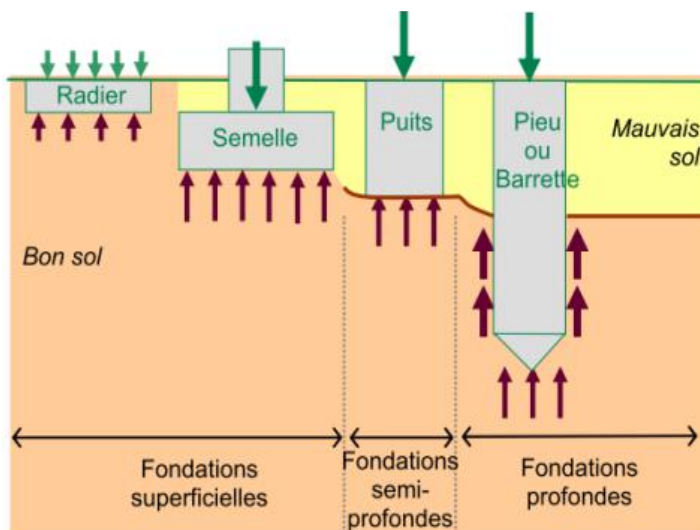
-Figure 5-3: les types de fondations-
