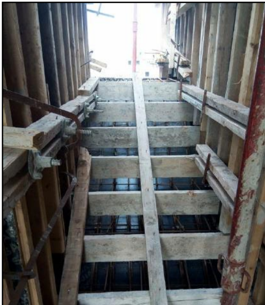
-Figure 7-6 : Coffrage d'escalier-
