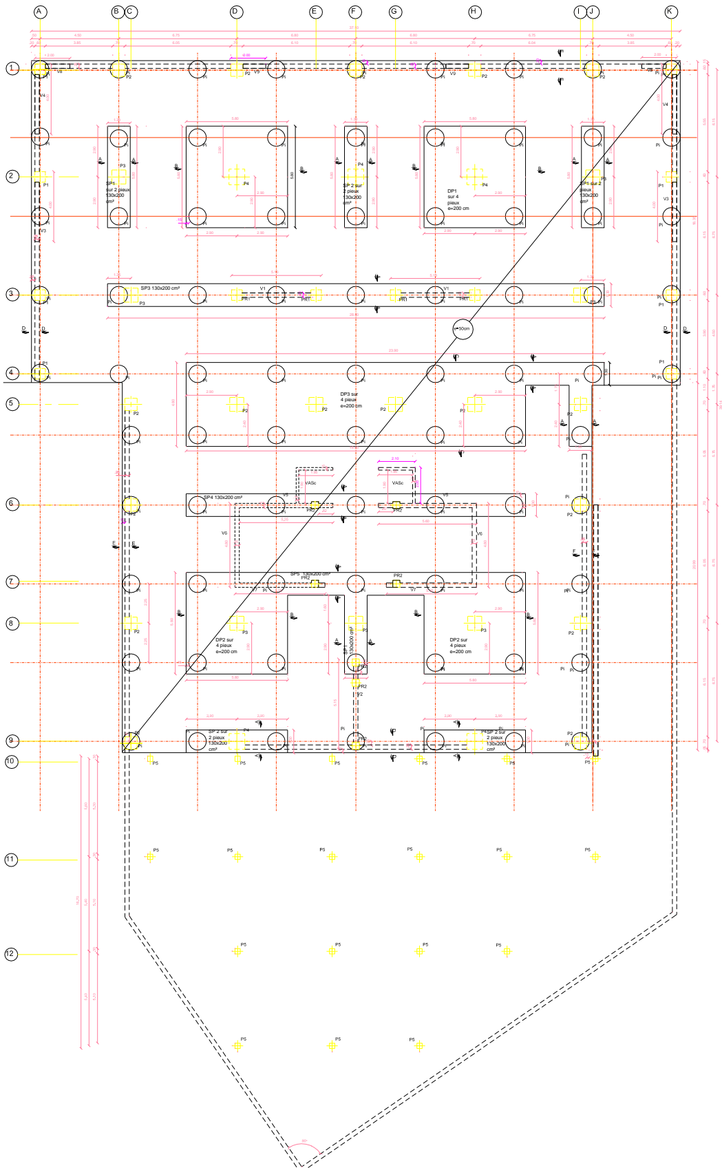
-Coffrage fondation sur pieux-
