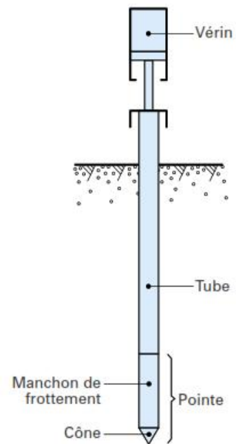
Figure 4-3 : Schéma de principe du pénétrromètre statique
