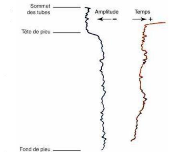
Figure 5-15 : Exemples d'enregistrement de l'amplitude et du temps sur un pieu
