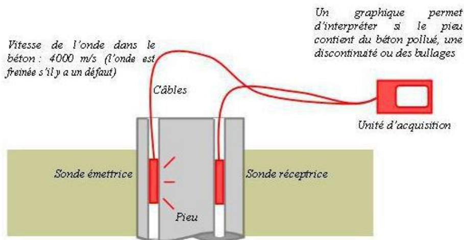
-Figure 5-7: Principe de l'essai de sonique-
