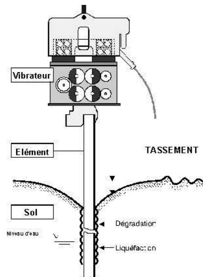
Figure 5-20: Le principe du fonçage par vibration
