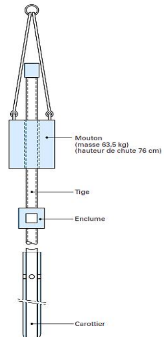
Figure 4-4 : Schéma de principe du SPT
