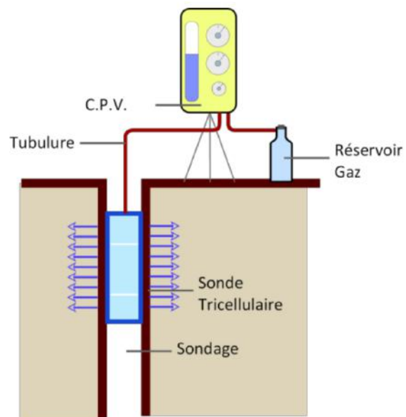
Figure 4-5 : Schéma de principe du pressiométrique
